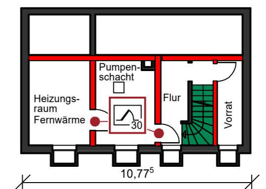
GRUNDRISS KELLERGESCHOSS
