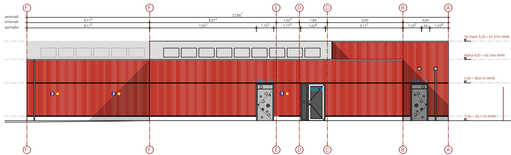
ANSICHT OST
