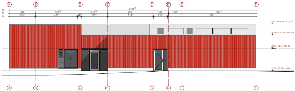
ANSICHT WEST
