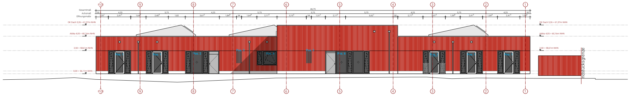
ANSICHT NORD
