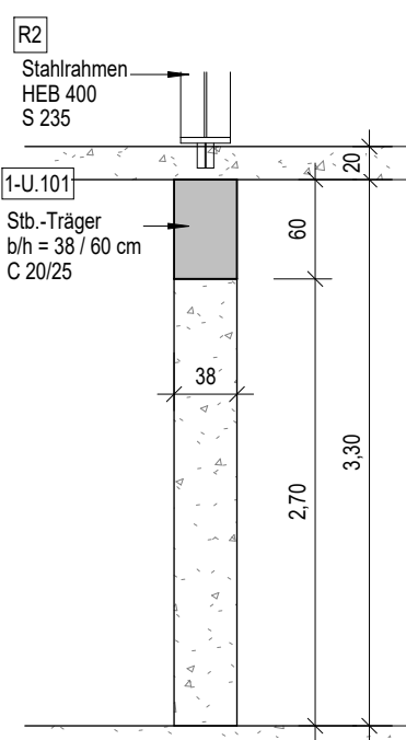
Schnitt U-1 - M.: 1 : 50
