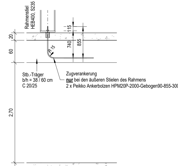
Schnitt U-2 - M.: 1 : 50
