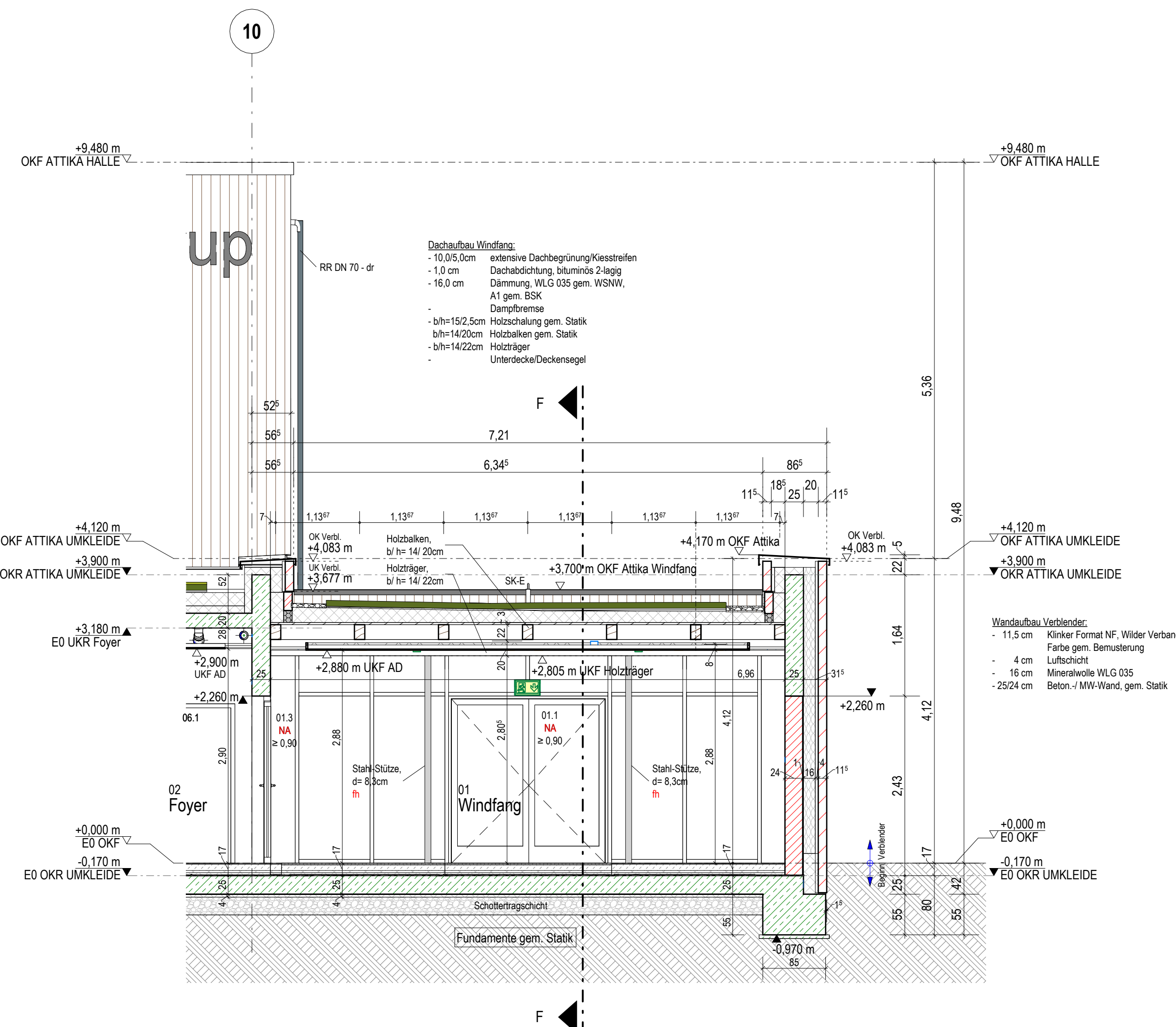
Schnitt E-E M. 1 : 50
