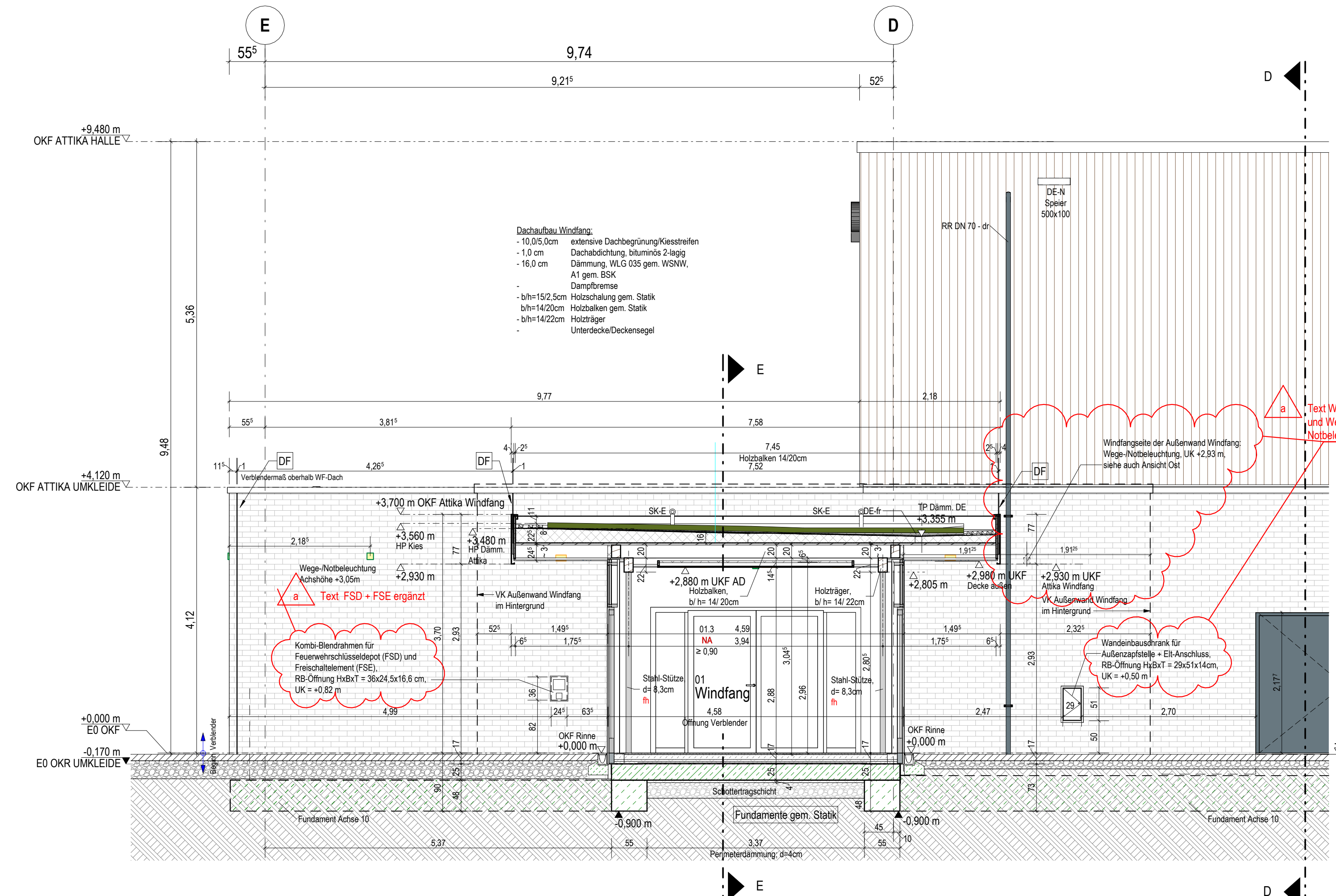
Schnitt F-F M. 1 : 50
