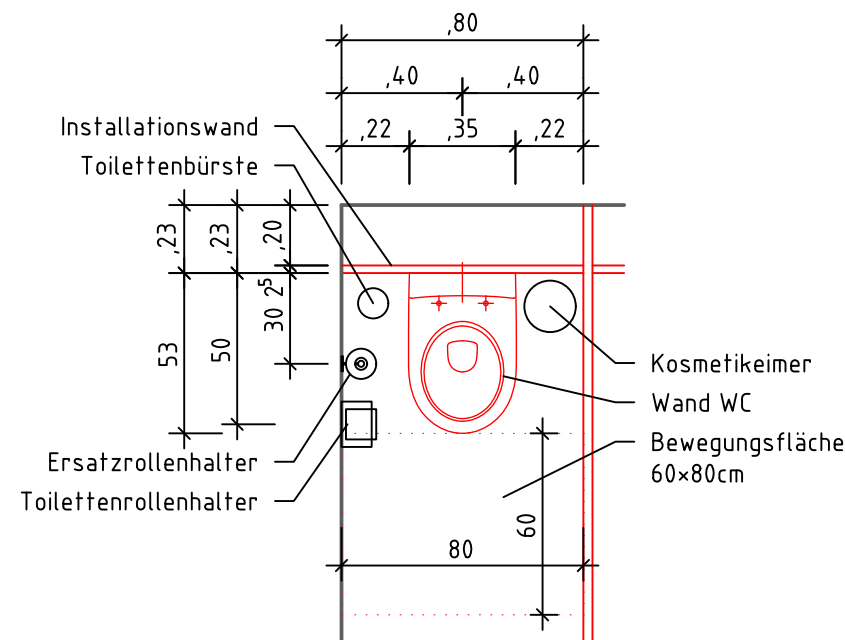
Anordnung WC-Zubehör 1:25
