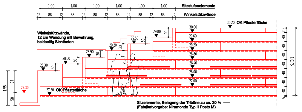
südliches Tribünenende, Ansicht von vorne, M= 1:50
