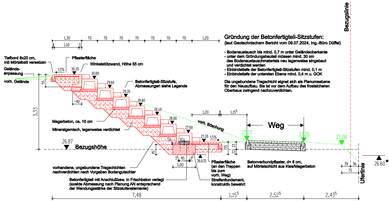
Geländeschnitt S4, M= 1:50
