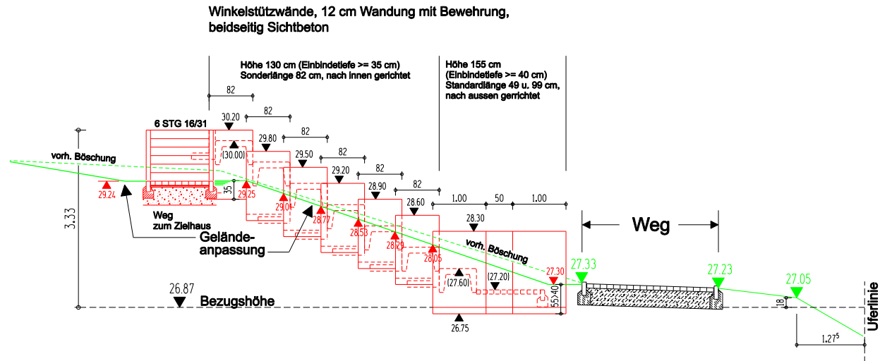
südliches Tribünenende, Ansicht von der Seite, M= 1:50
