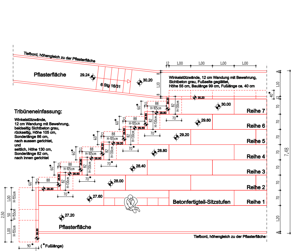
südliches Tribünenende - Draufsicht, M= 1:50
