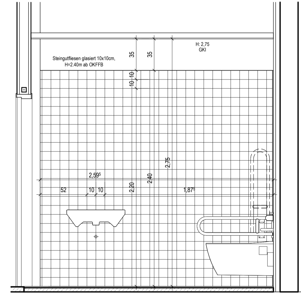
Beh. WC R7-4-113 Ansicht B M. 1:20
