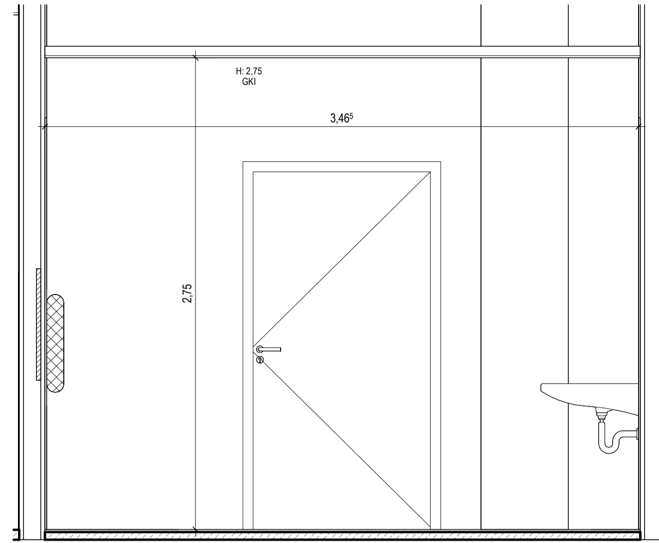
Beh. WC R7-4-113 Ansicht A M. 1:20
