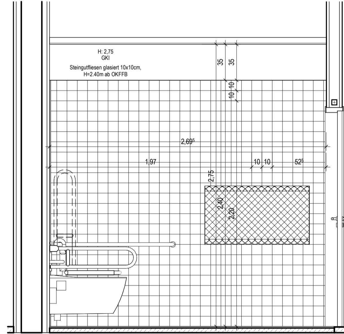
Beh. WC R7-4-113 Ansicht D M. 1:20
