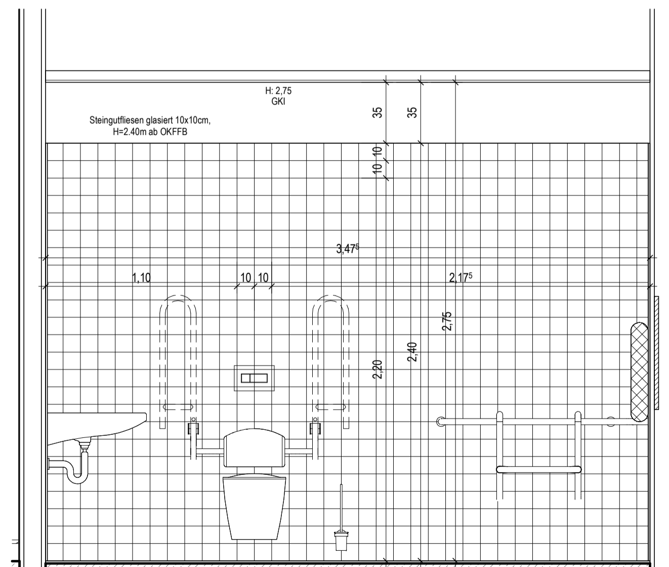
Beh. WC R7-4-113 Ansicht C M. 1:20
