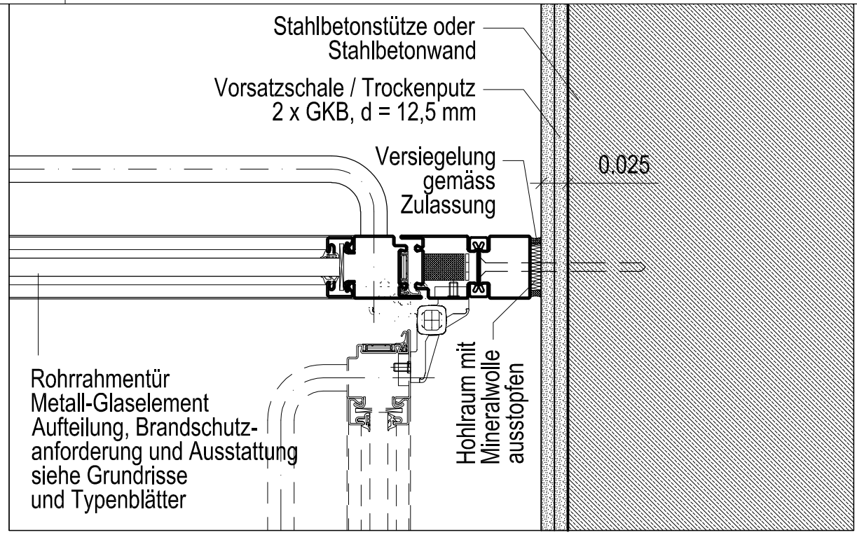
Wandanschluss Massivwand (F30)
