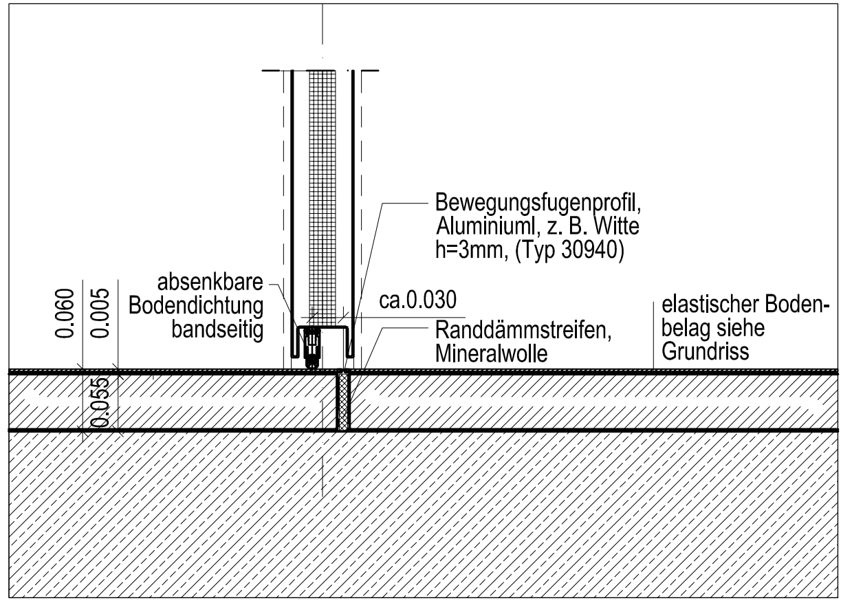
unterer Anschluss
