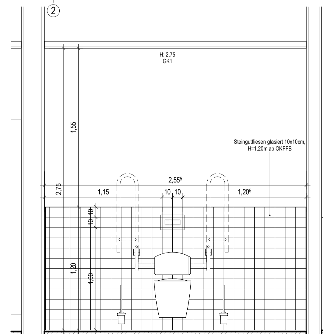
Beh. WC R7-1-117 Ansicht C M. 1:20
