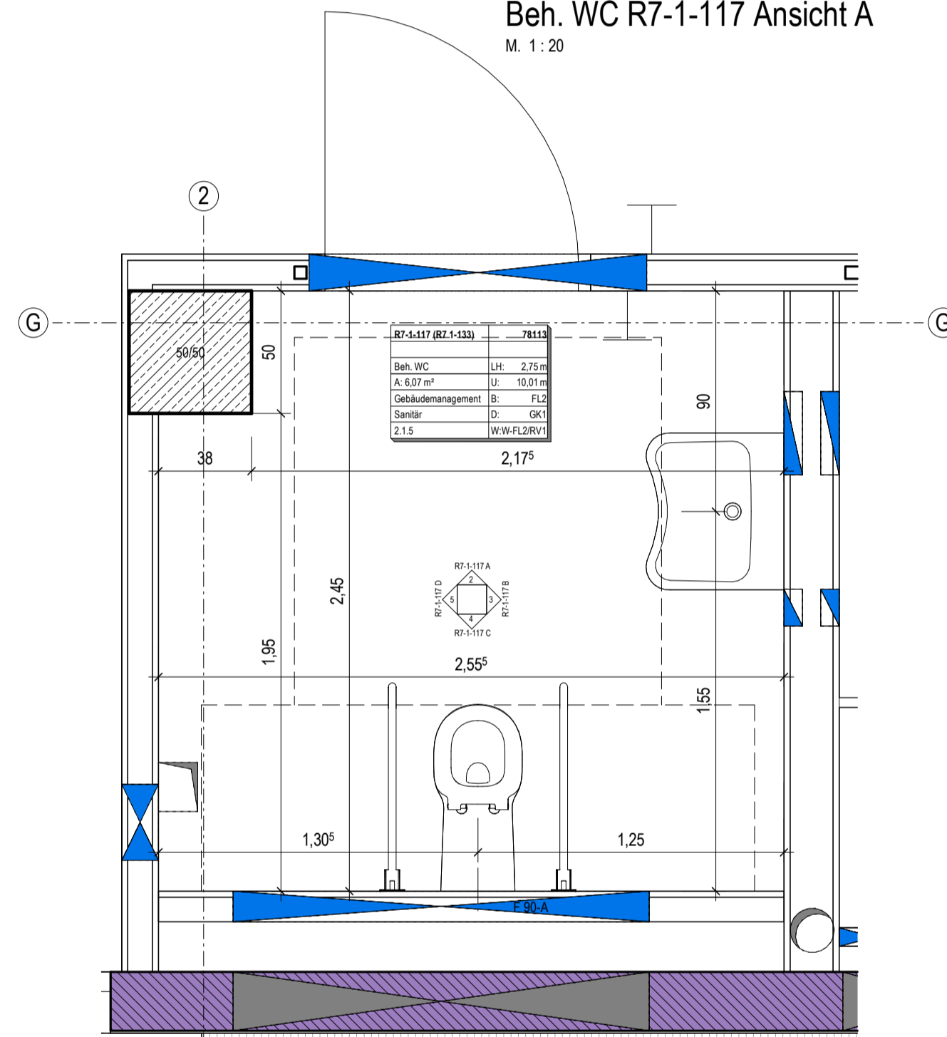
Grundriss Dusche Pers. R7-1-117 M. 1:20
