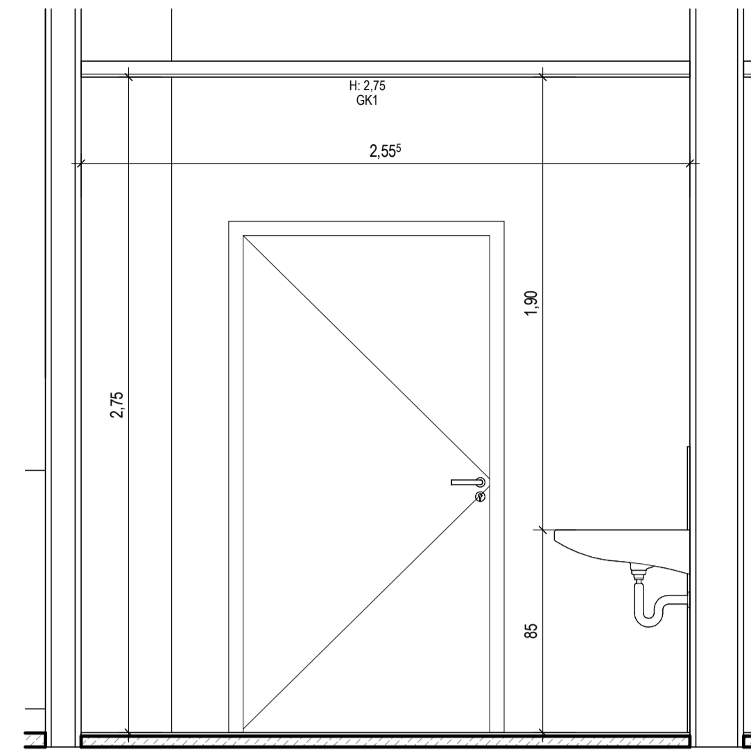
Beh. WC R7-1-117 Ansicht A M. 1:20
