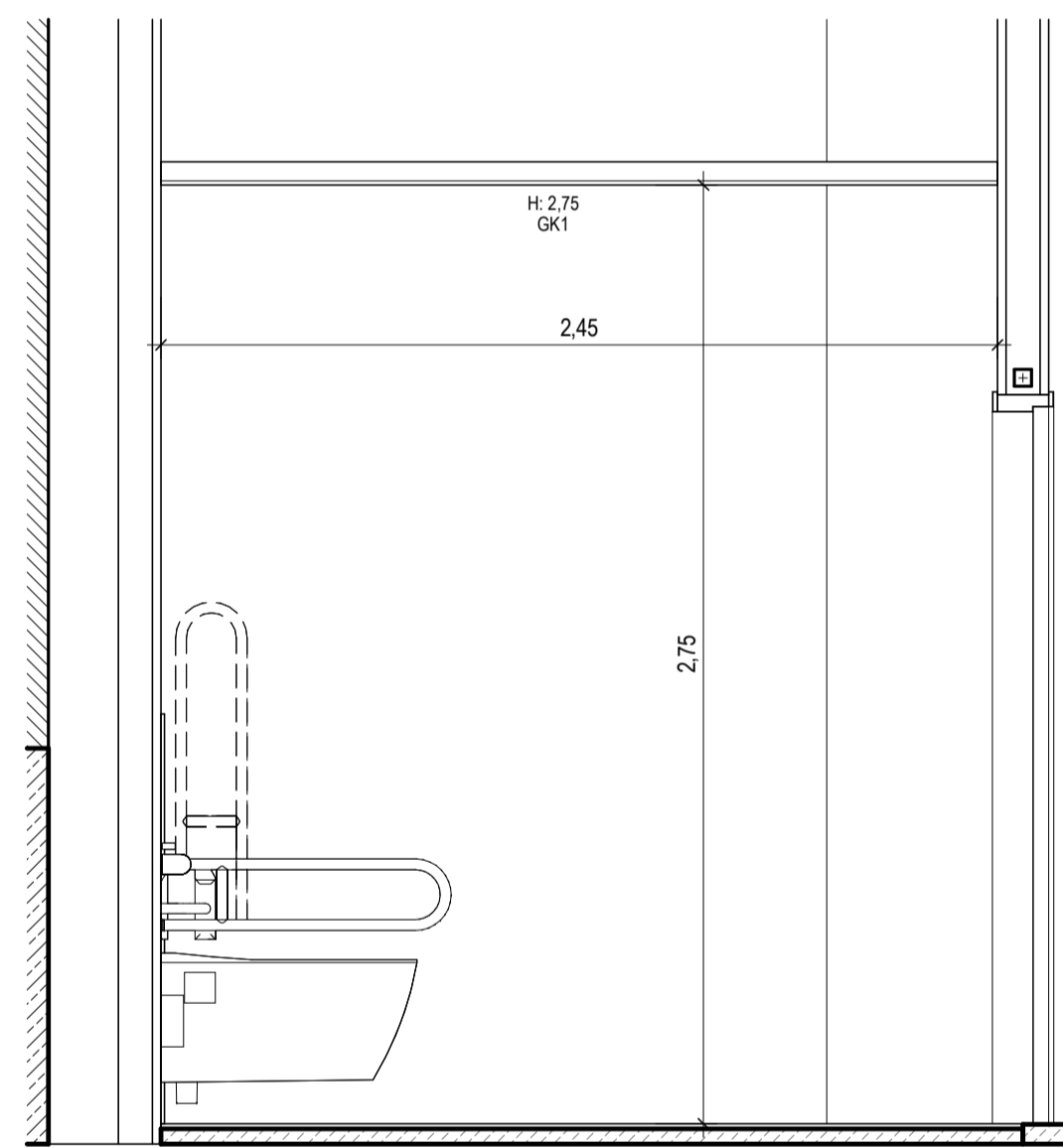
Beh. WC R7-1-117 Ansicht D M. 1:20
