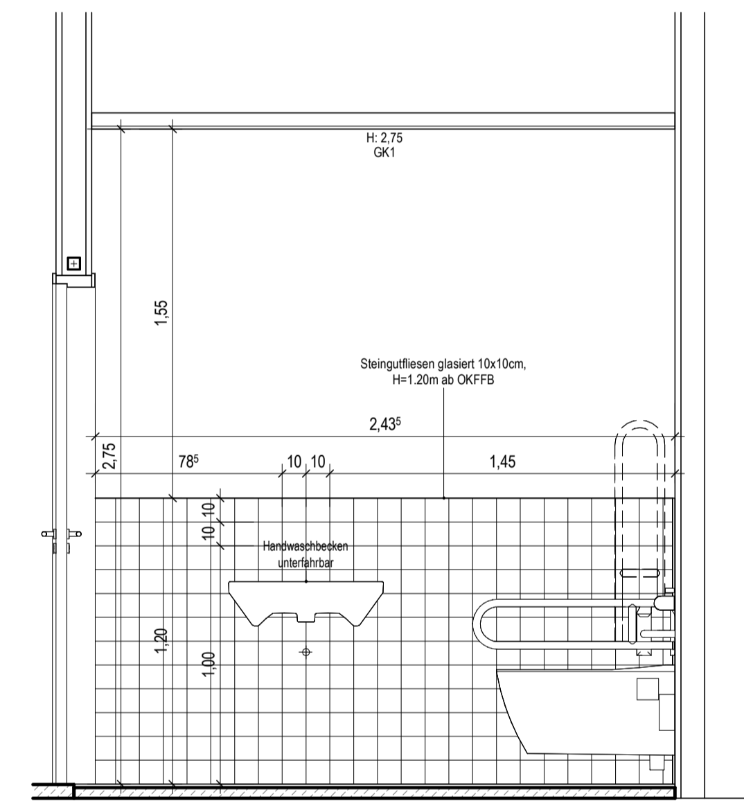
Beh. WC R7-1-117 Ansicht B M. 1:20
