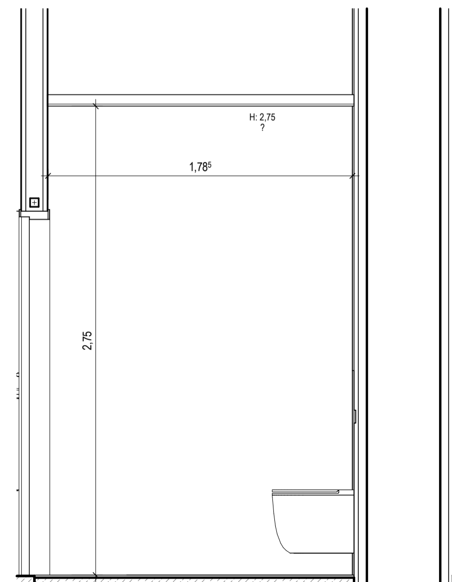
WC R7-4-103 Ansicht C M. 1:20
