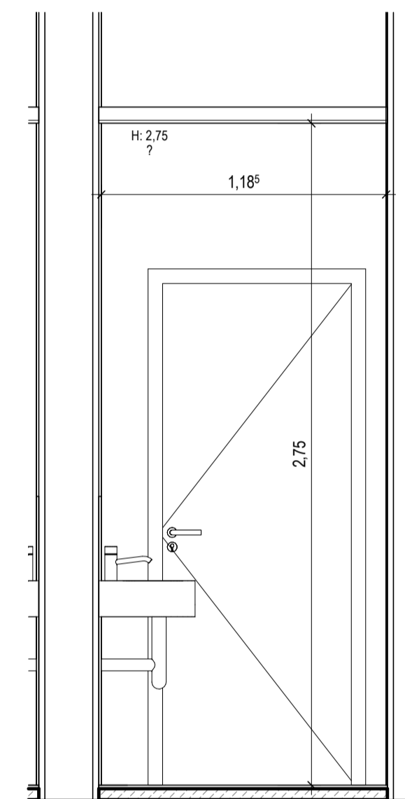
WC R7-4-103 Ansicht B M. 1:20
