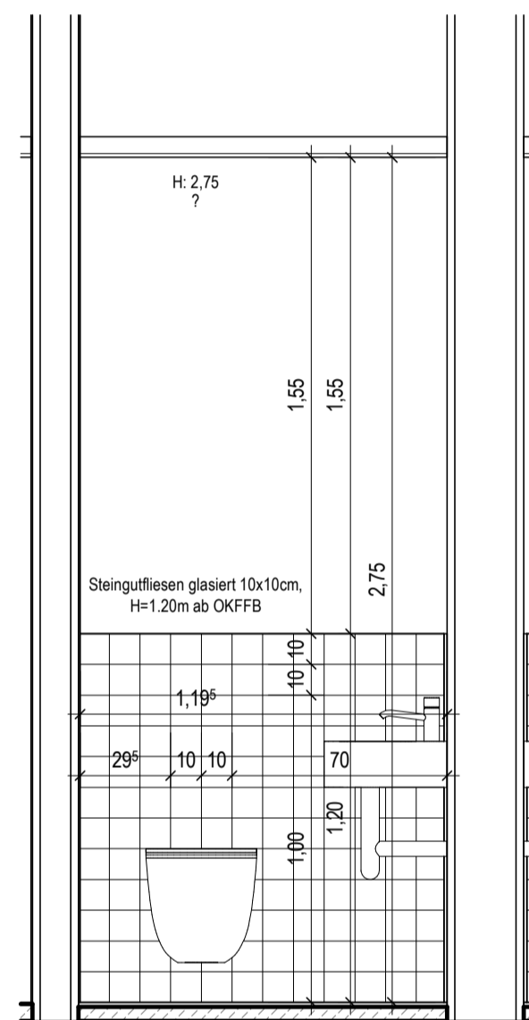
WC R7-4-103 Ansicht D M. 1:20
