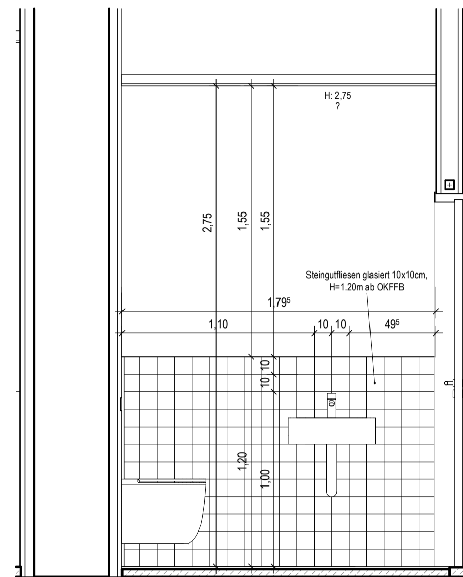
WC R7-4-103 Ansicht A M. 1:20
