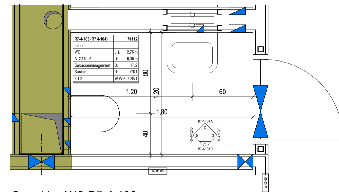
Grundriss WC R7-4-103 M. 1:20
