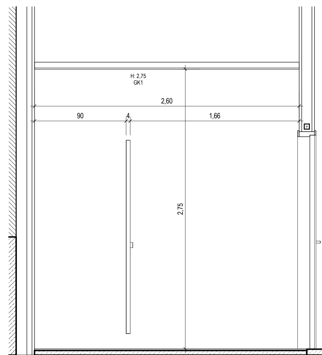
WC R7-1-116 Ansicht D M. 1:20
