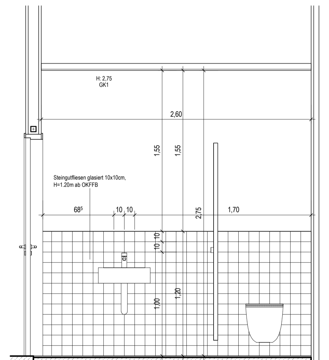
WC R7-1-116 Ansicht B M. 1:20
