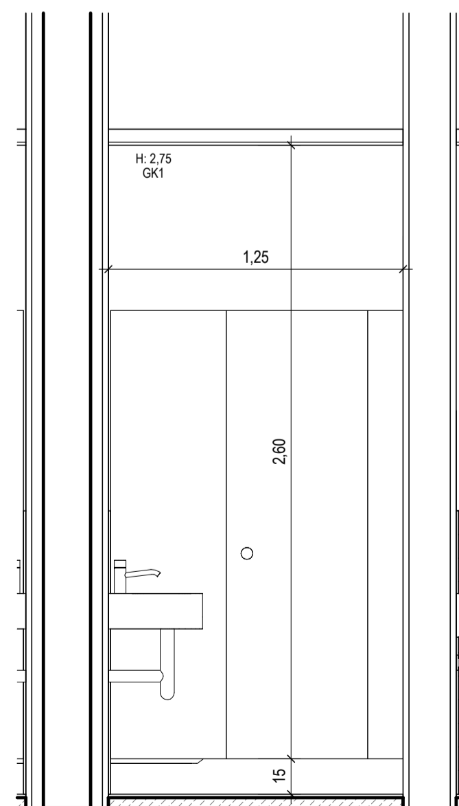
WC R7-1-116 Ansicht C M. 1:20
