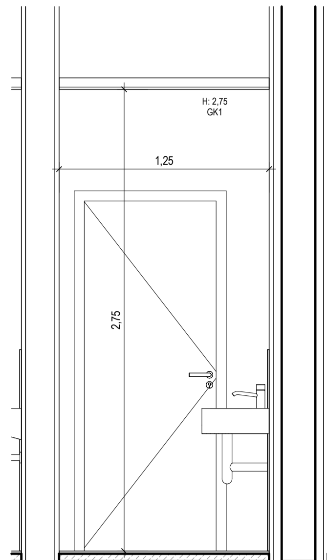
WC R7-1-116 Ansicht A M. 1:20
