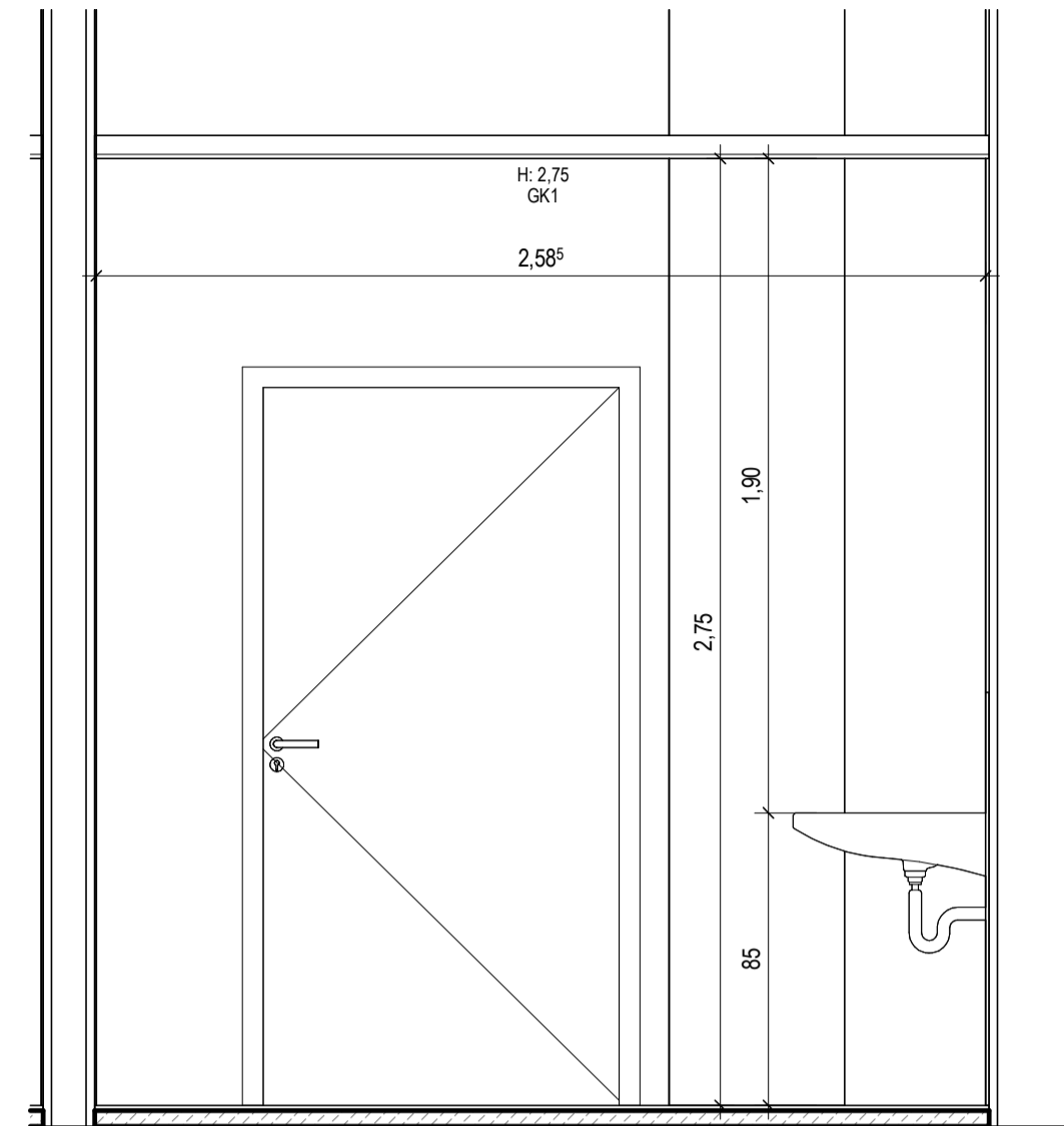
Beh. WC R7-3-113 Ansicht A M. 1 : 20
