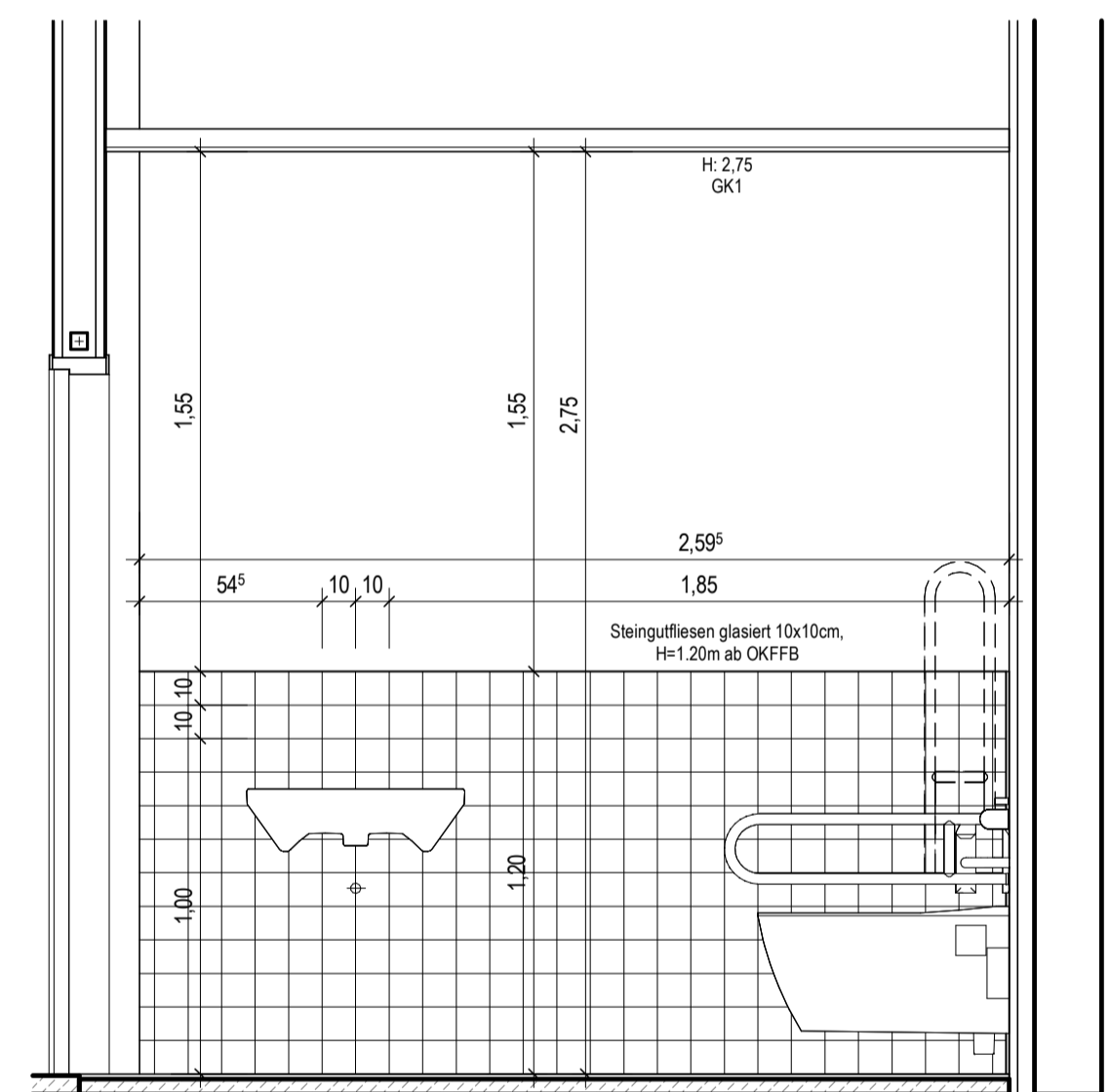
Beh. WC R7-3-113 Ansicht B M. 1 : 20
