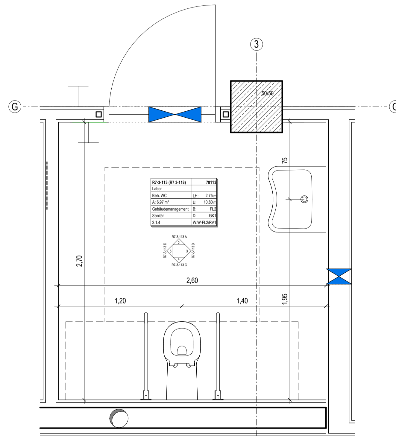
Grundriss Beh. WC R7-3-113 M. 1 : 20
