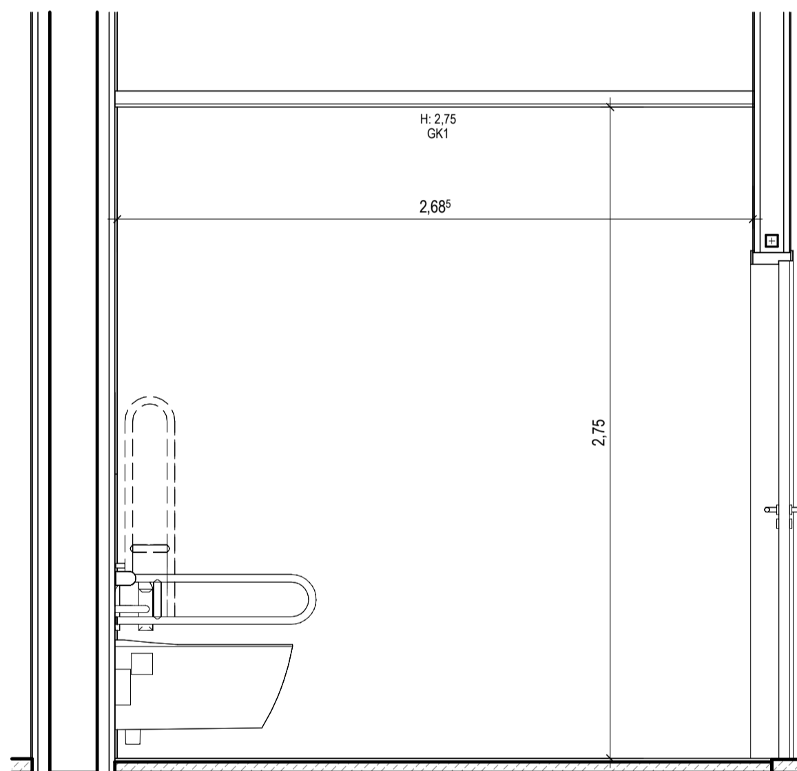
Beh. WC R7-3-113 Ansicht D M. 1 : 20
