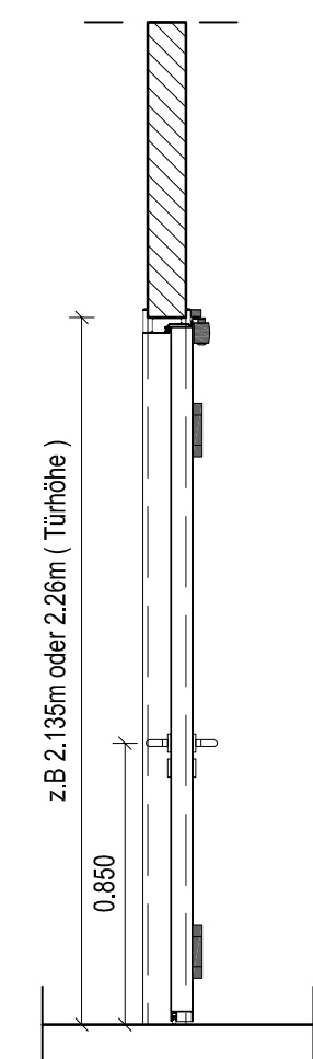
Schnitt
