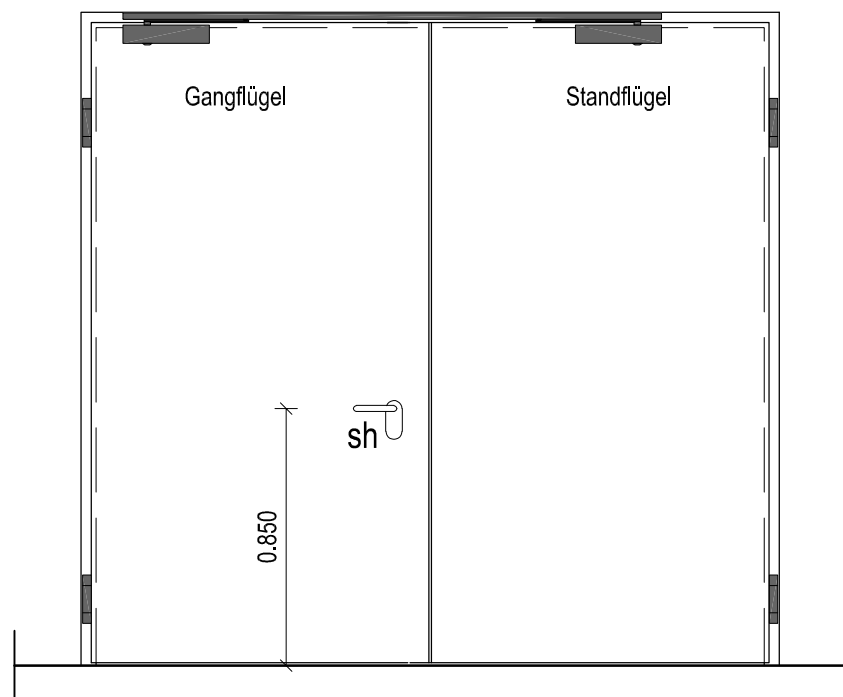
Ansicht Bandseite
