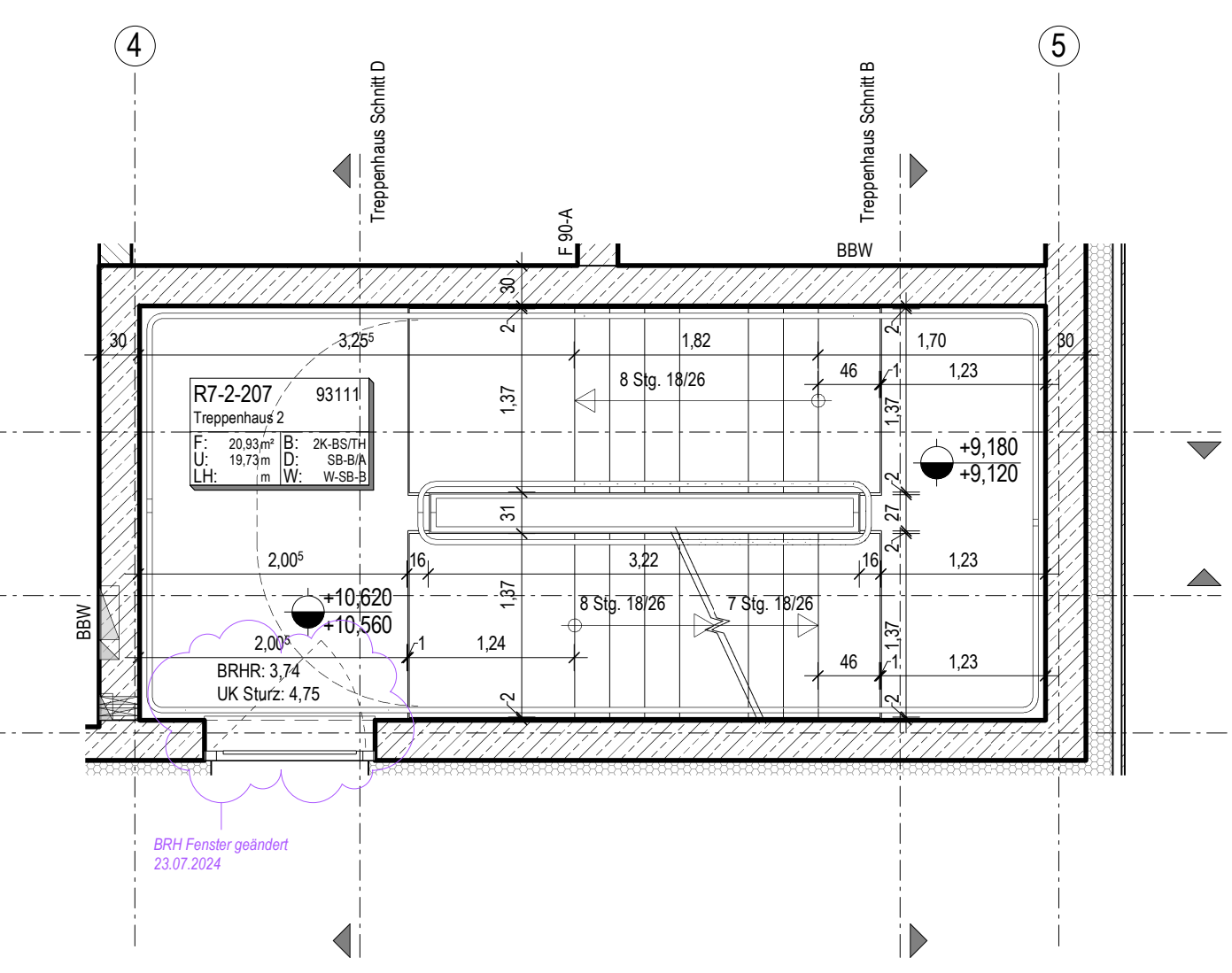
Grundriss 2OG Zwischengeschoss
