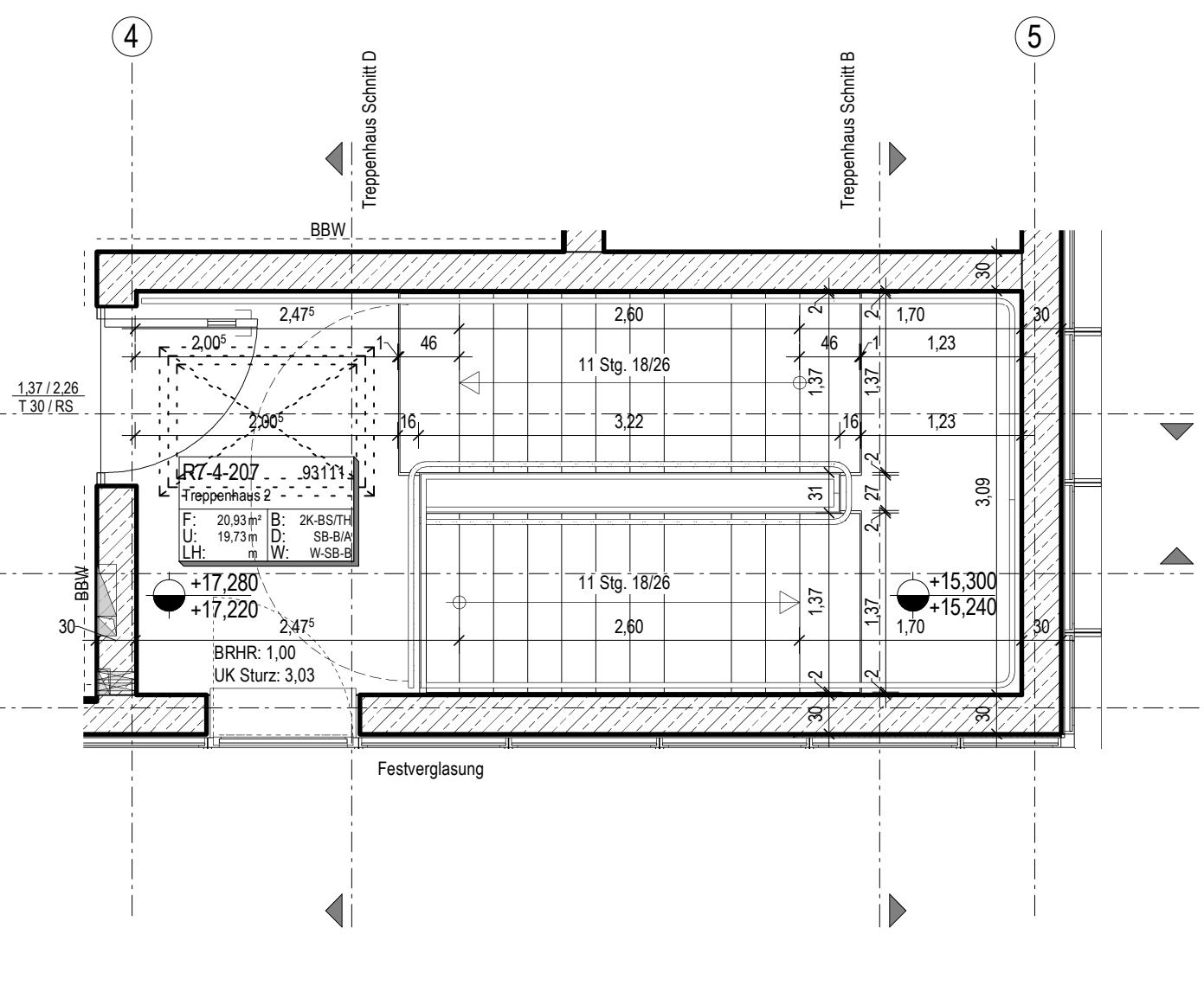
Grundriss 4OG
