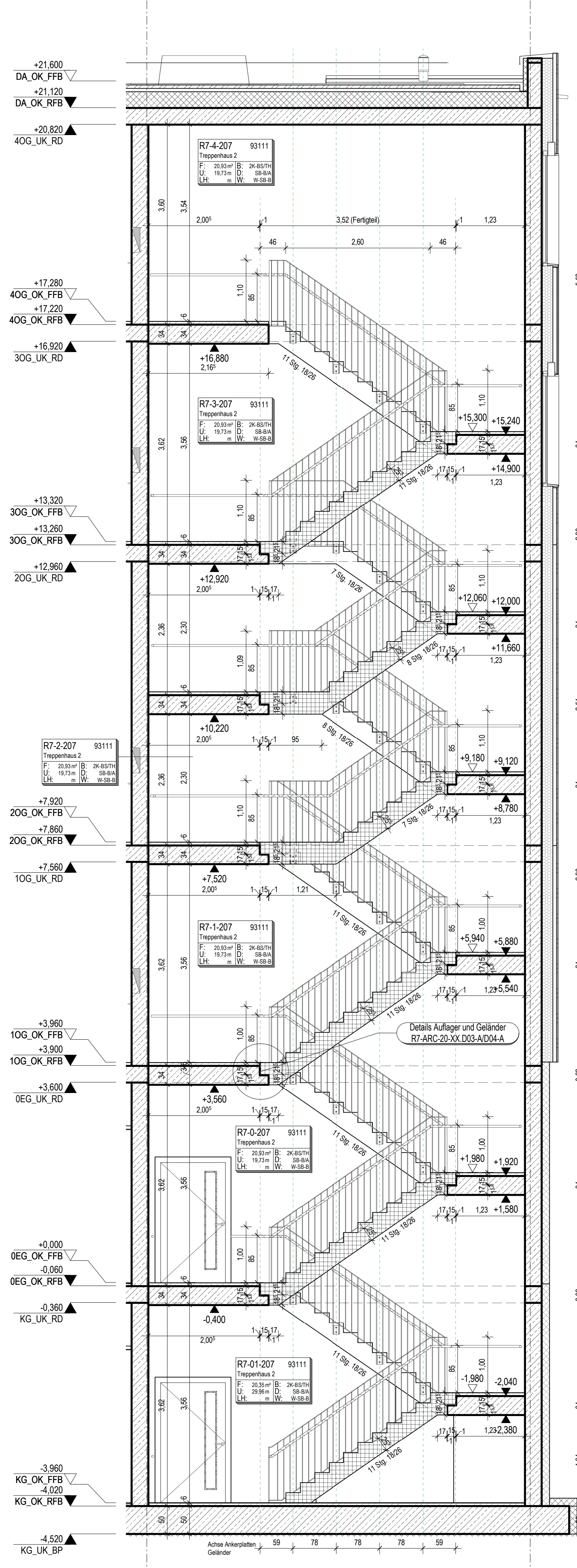
Treppenhaus Schnitt A
