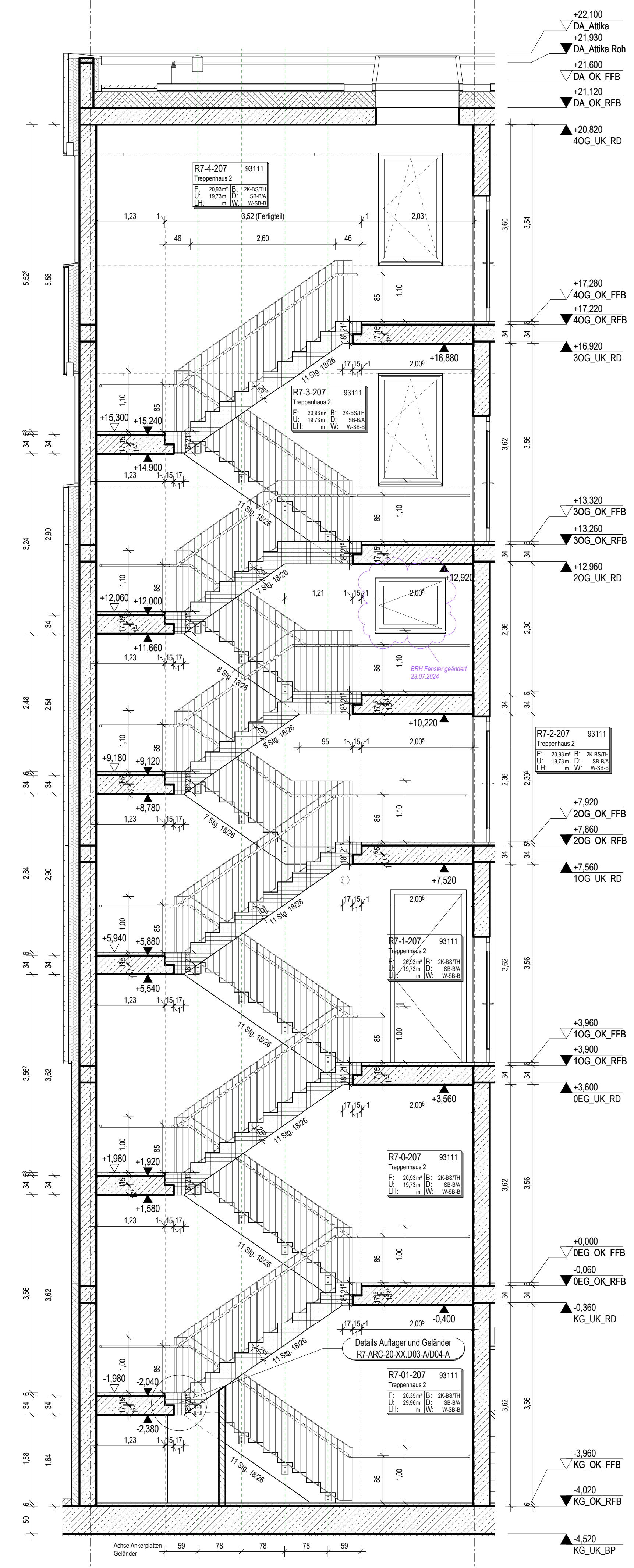
Treppenhaus Schnitt C
