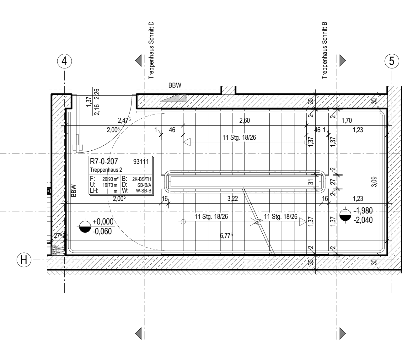
Grundriss EG
