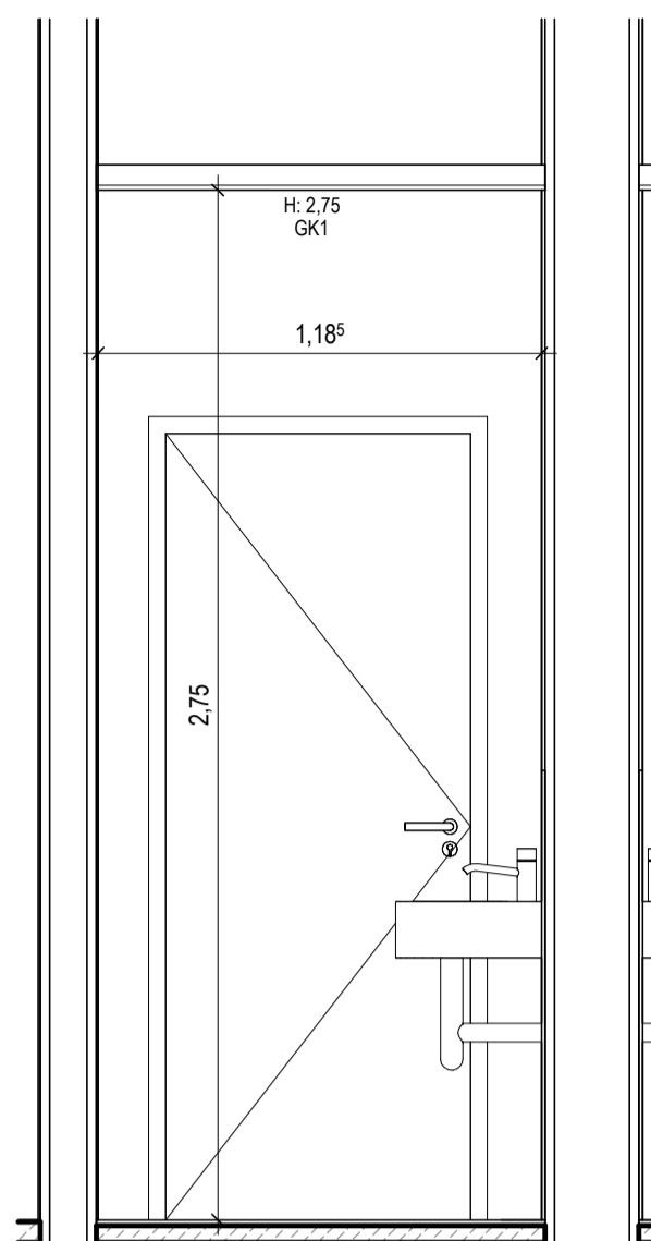
WC R7-3-115 Ansicht A M. 1:20
