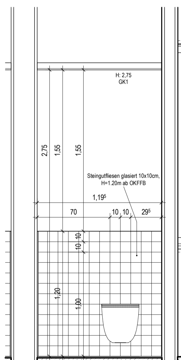
WC R7-3-115 Ansicht C M. 1:20
