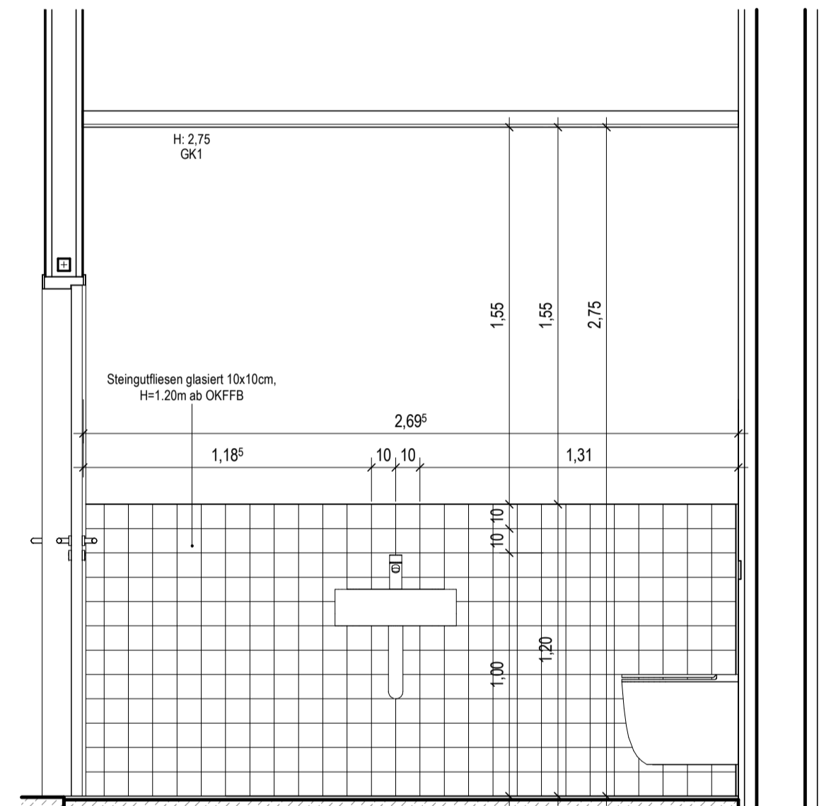
WC R7-3-115 Ansicht B M. 1:20
