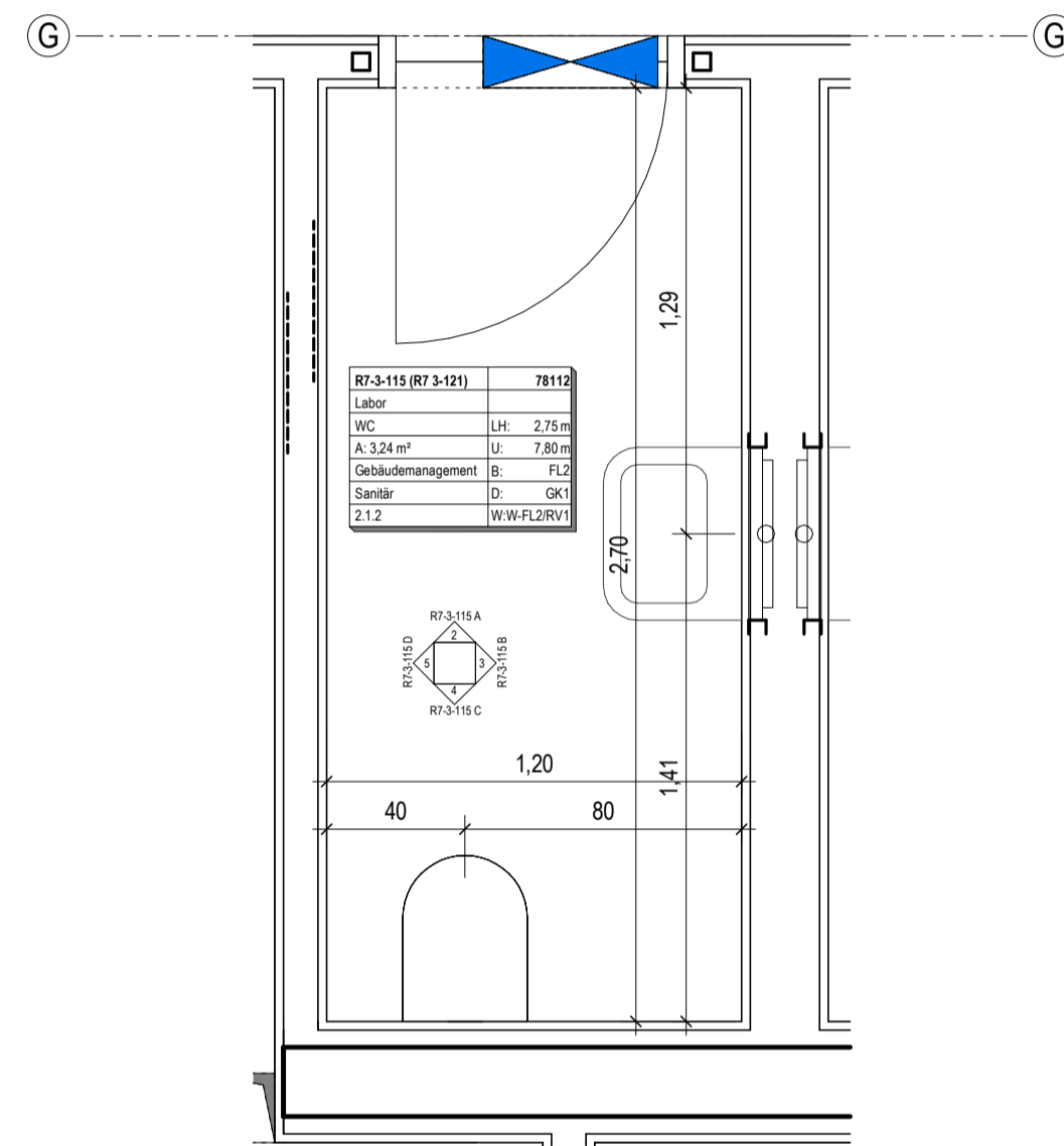
Grundriss WC R7-3-115 M. 1:20
