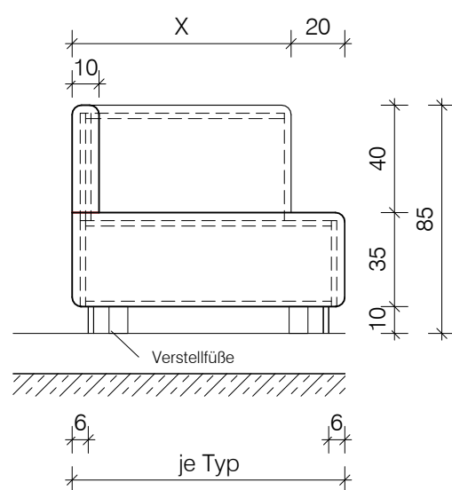
Schnitt B-B
