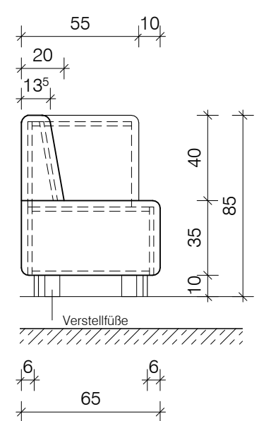
Schnitt A-A
