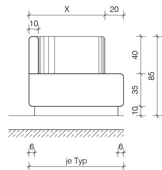
Schnitt C-C
