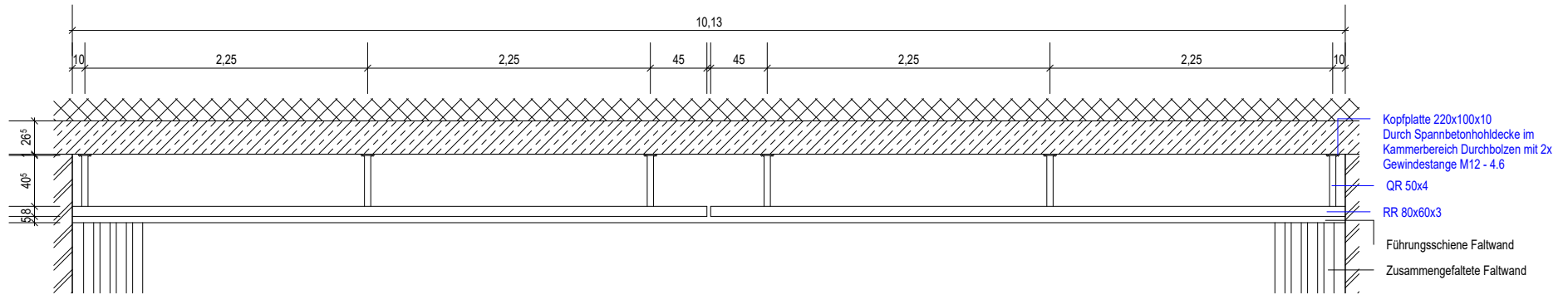
Schnitt längs Aufhängung Falte wand M: 1:50
