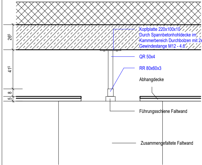
Schnitt quer Aufhängung Falte wand M: 1:25
