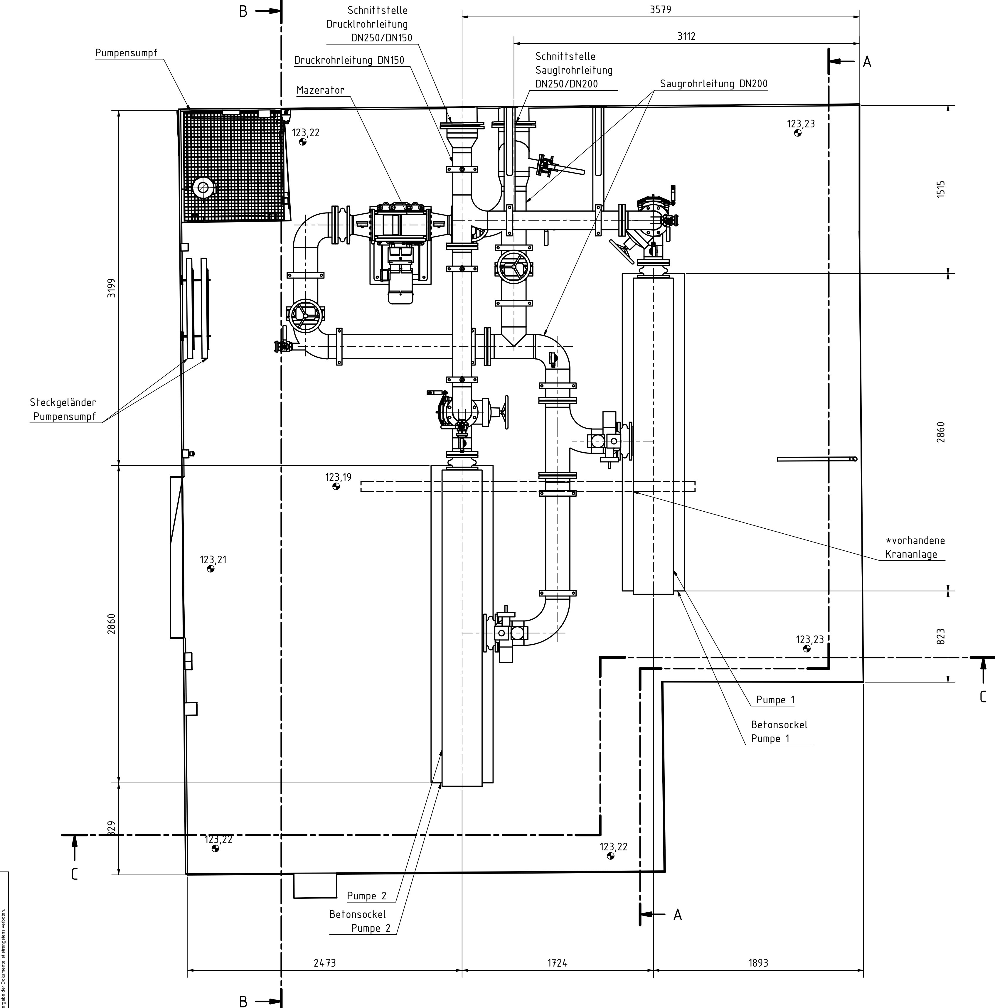
Maschinenkeller Grundriss
