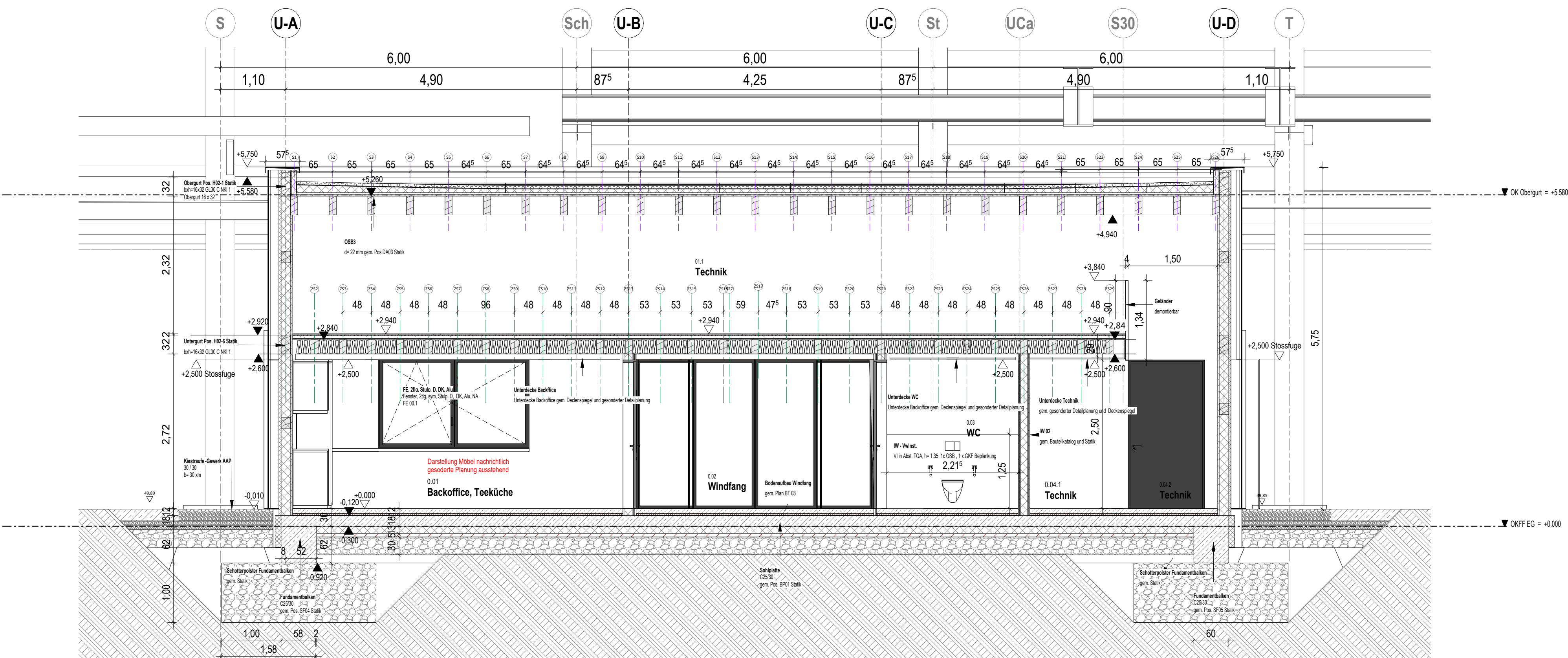
SC 1-1 LV Dachdecker
