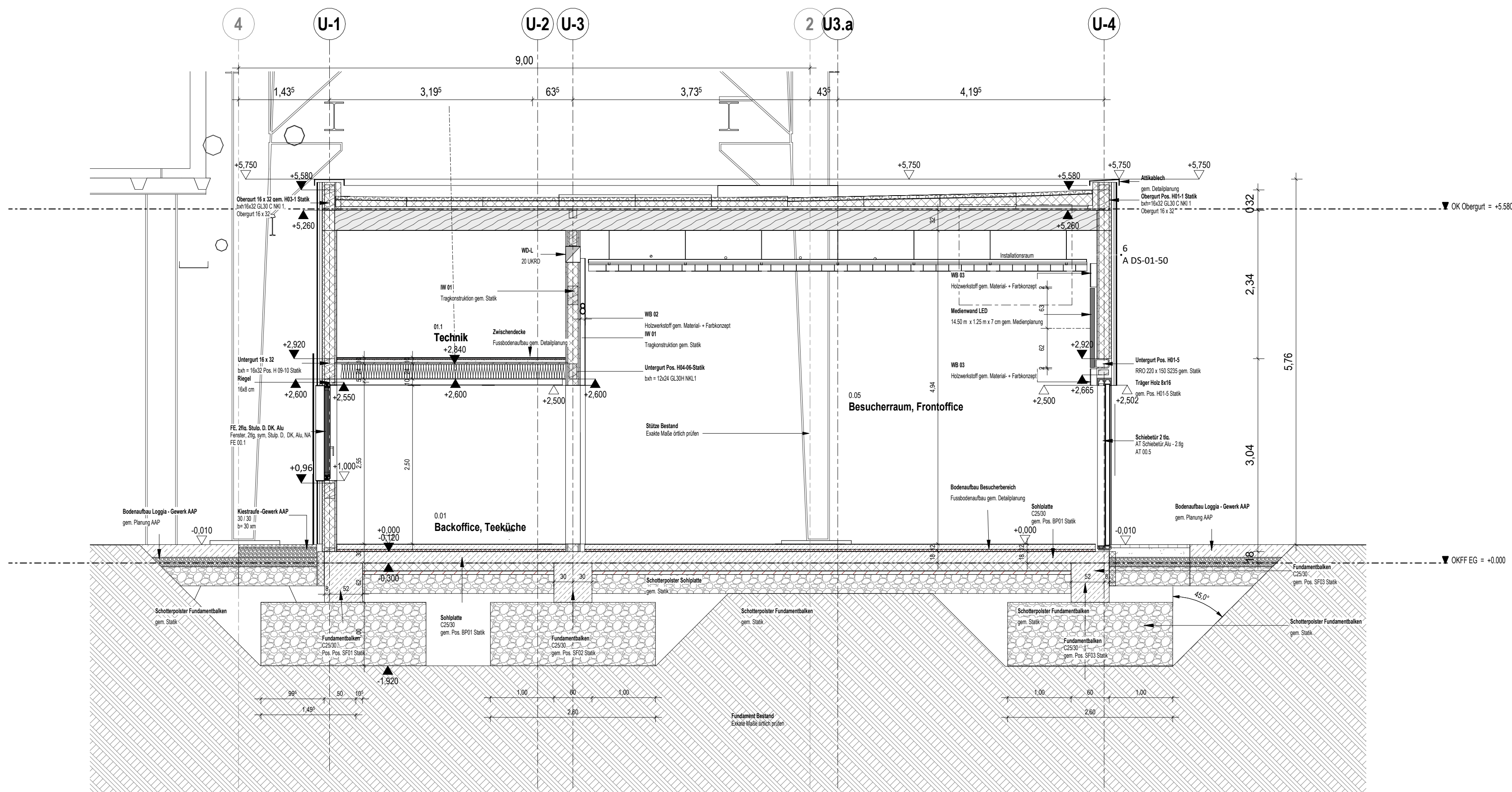
SC A-A LV Dachdecker
