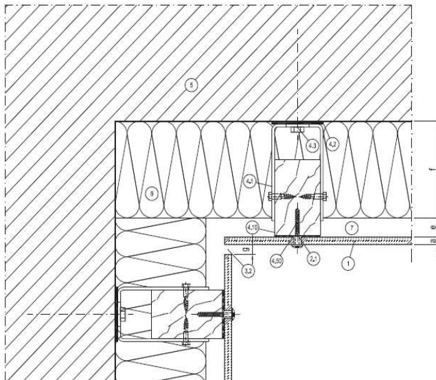
Horizontalschnitt h3.1
