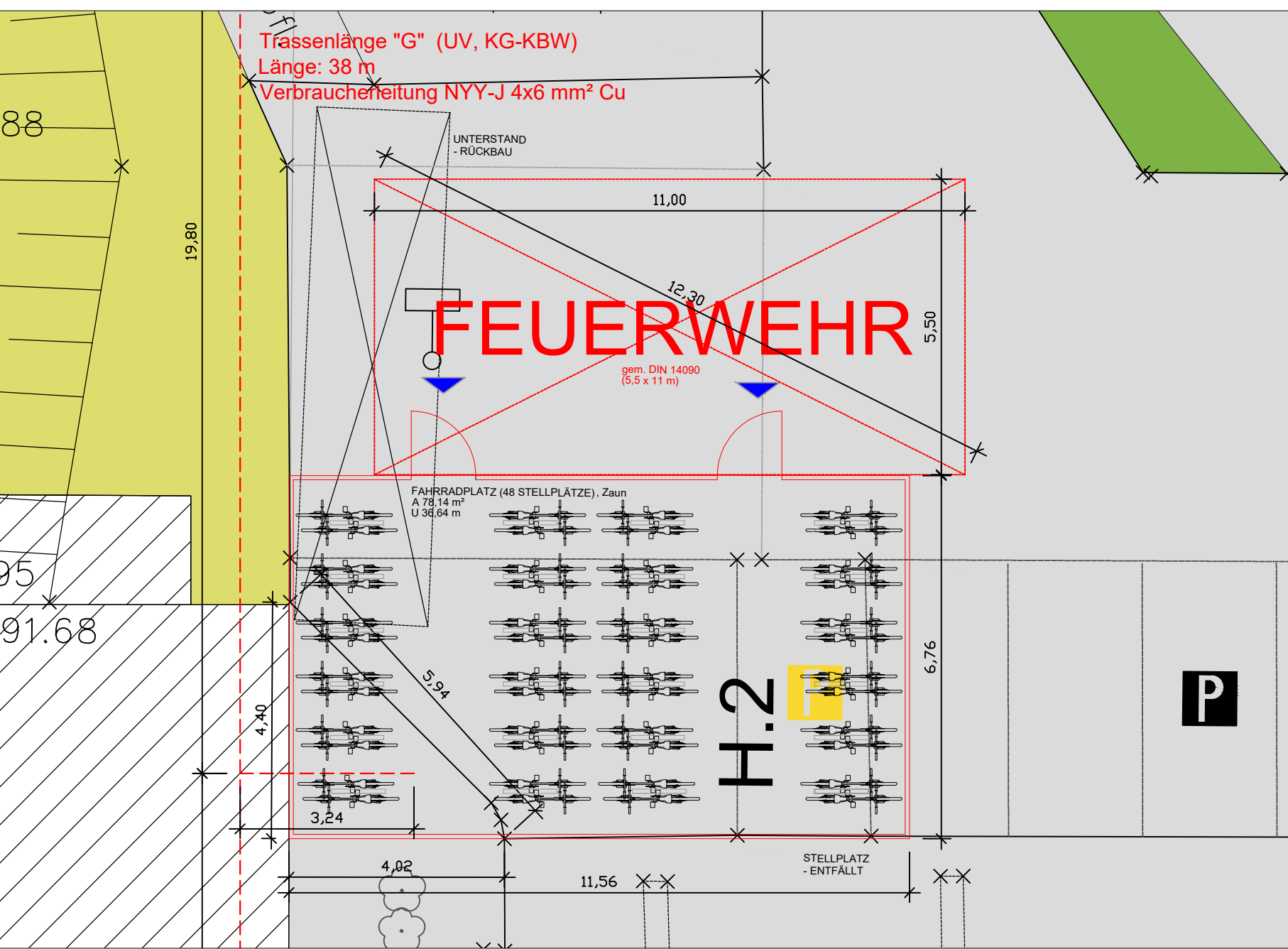
VARIANTE H.2 FAHRRADPLATZ 1:100
