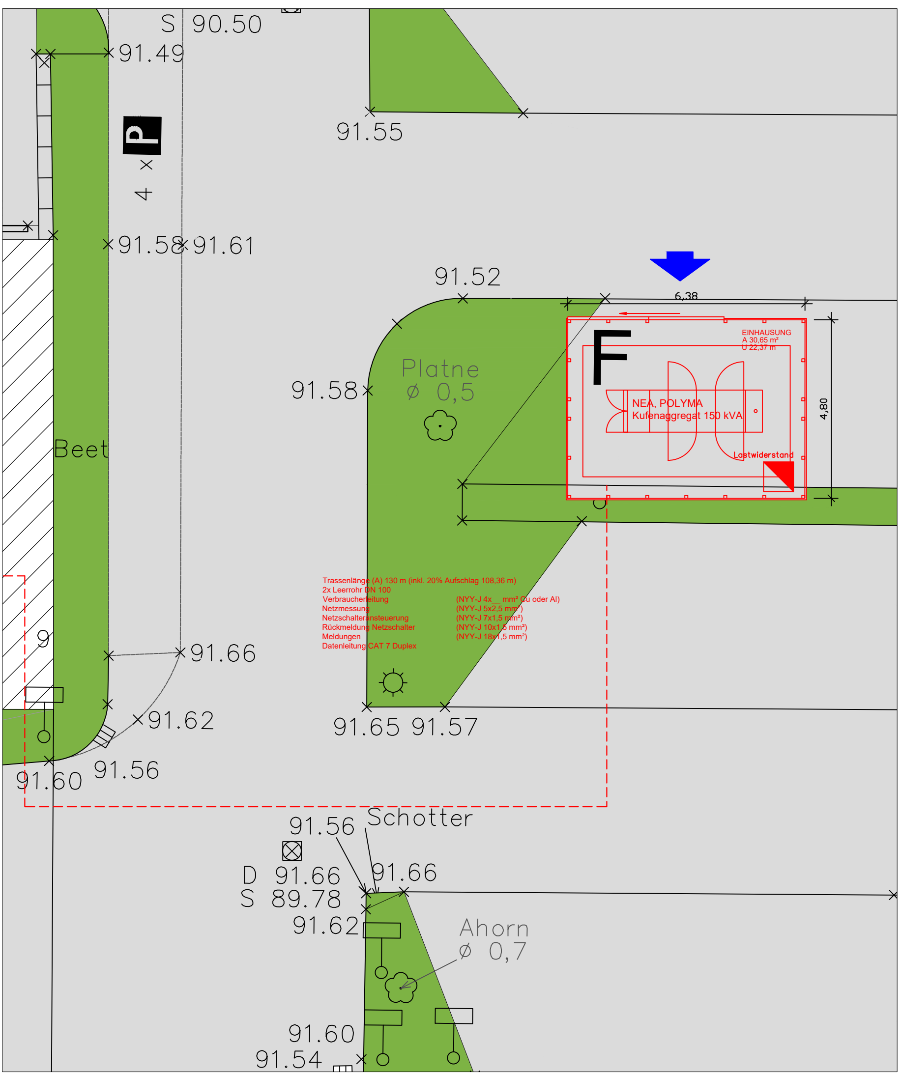
VARIANTE F 1:100
