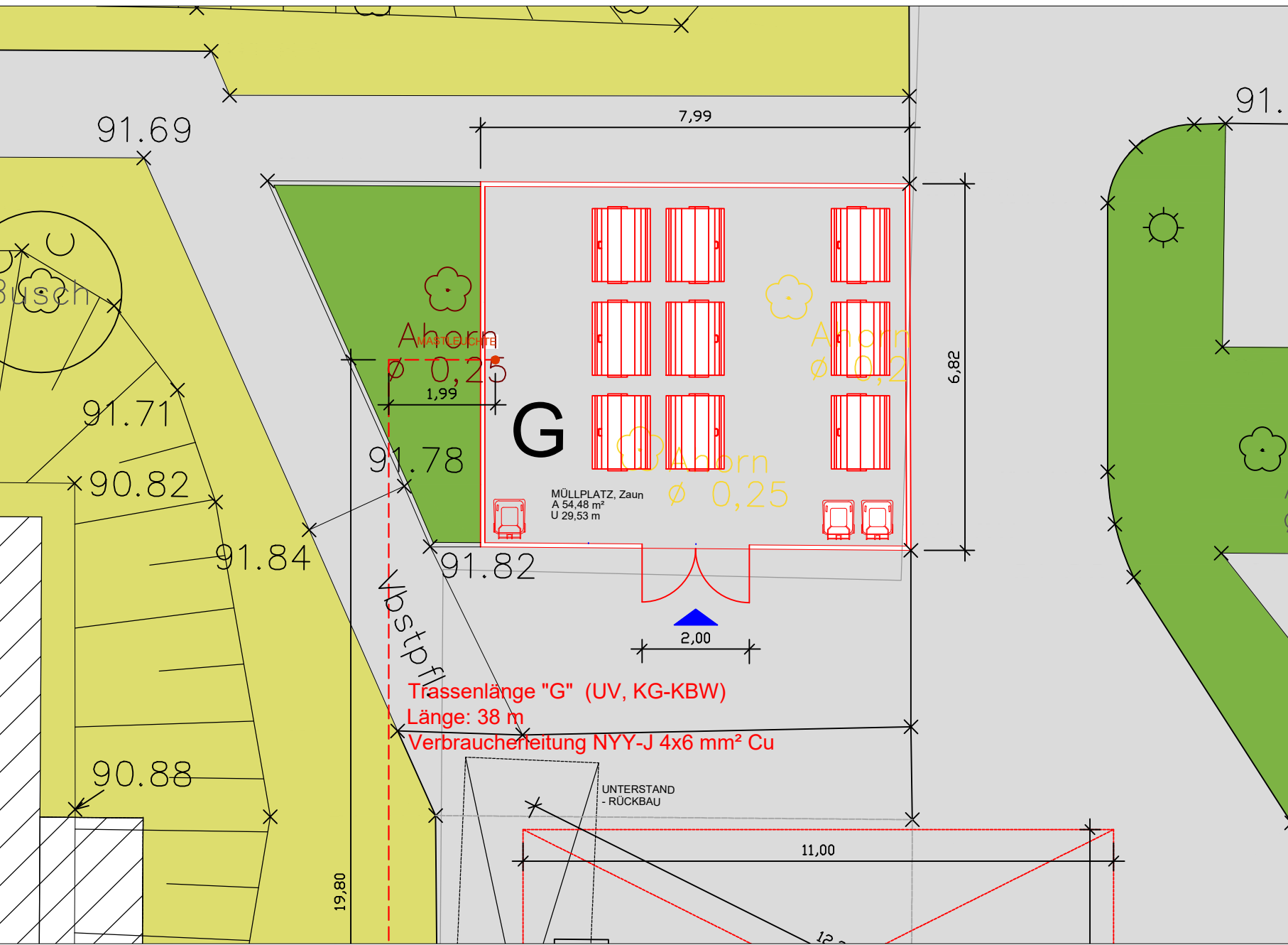
VARIANTE G - MÜLLPLATZ 1:100
