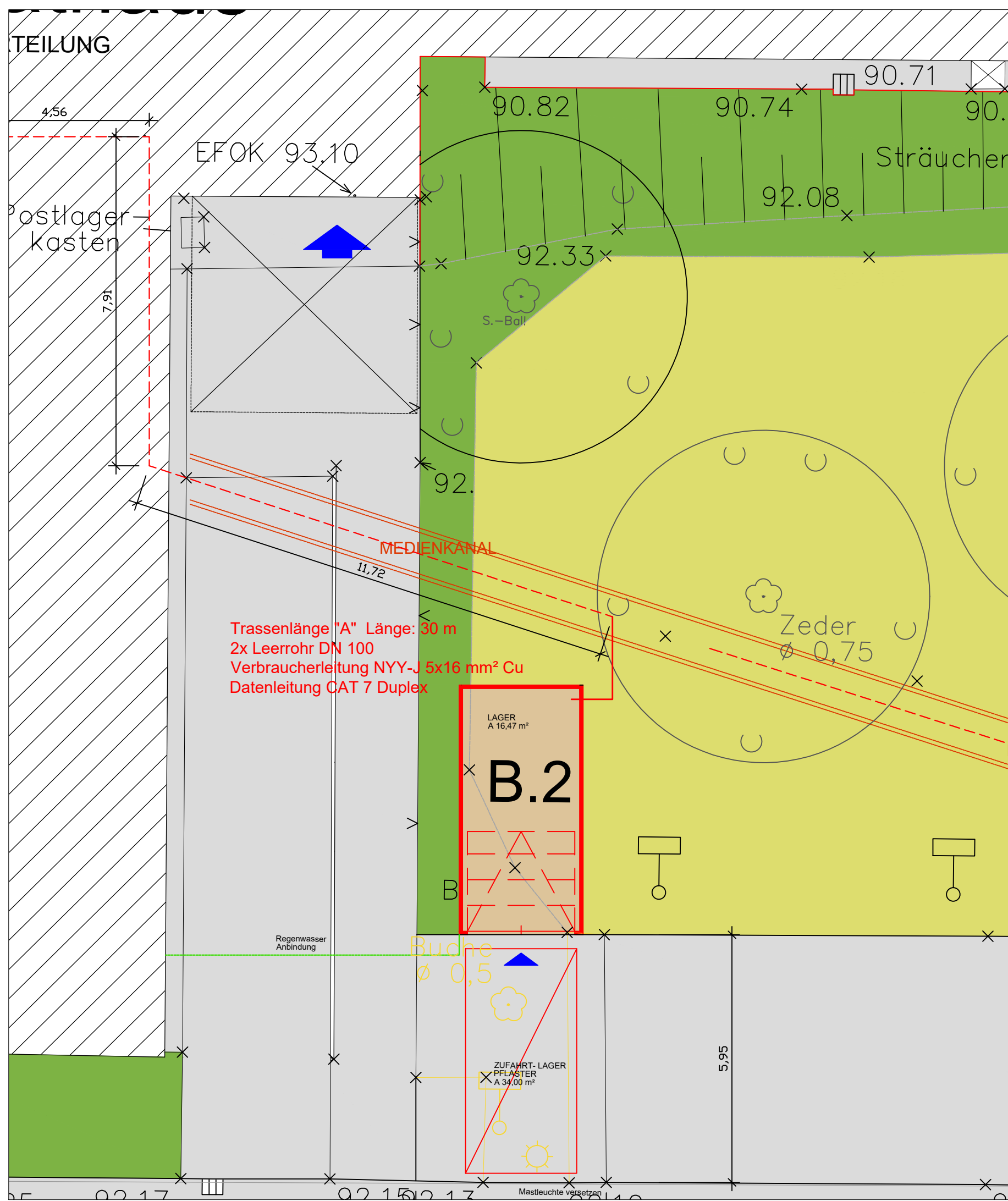
VARIANTE B.2 1:100
