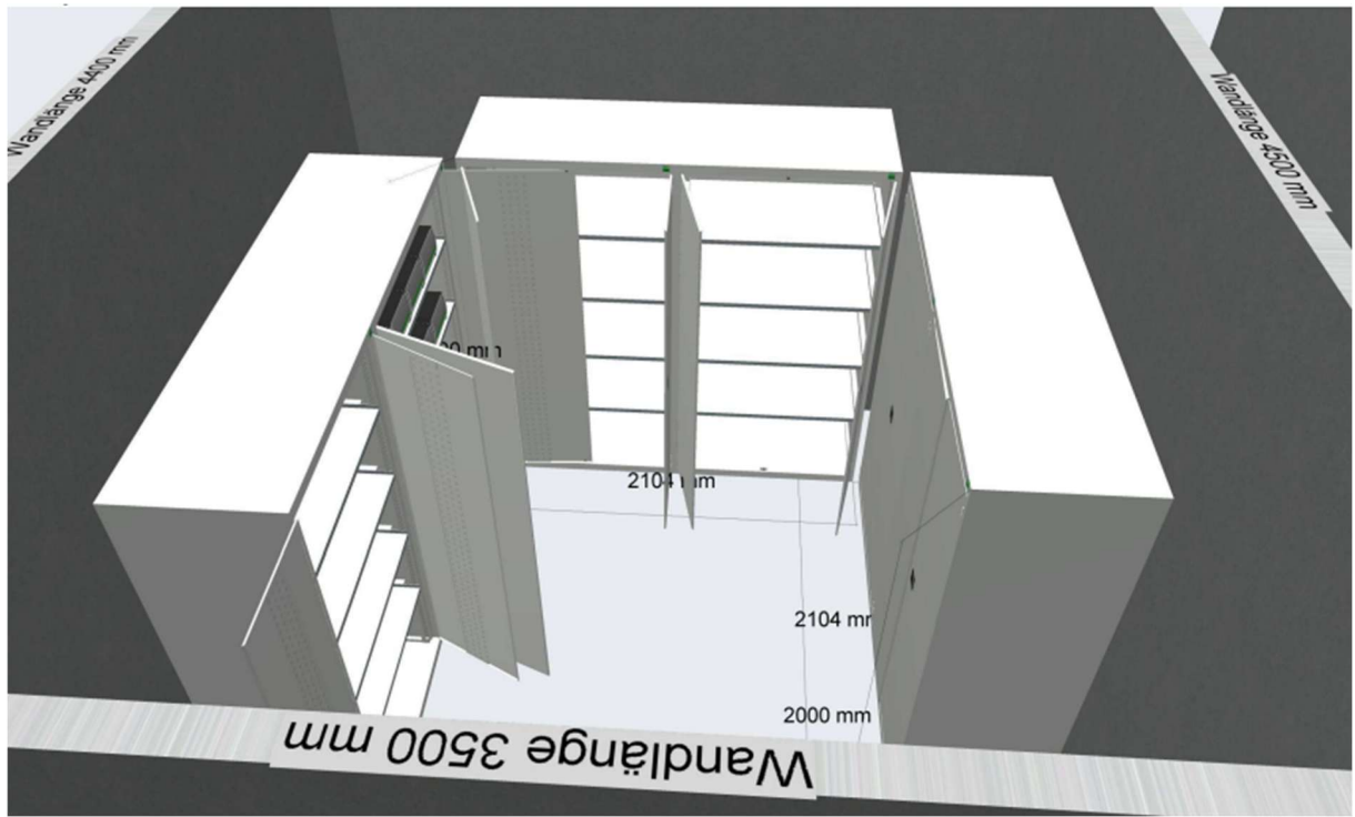
Bild 3: Systemschränke auf der Empore
