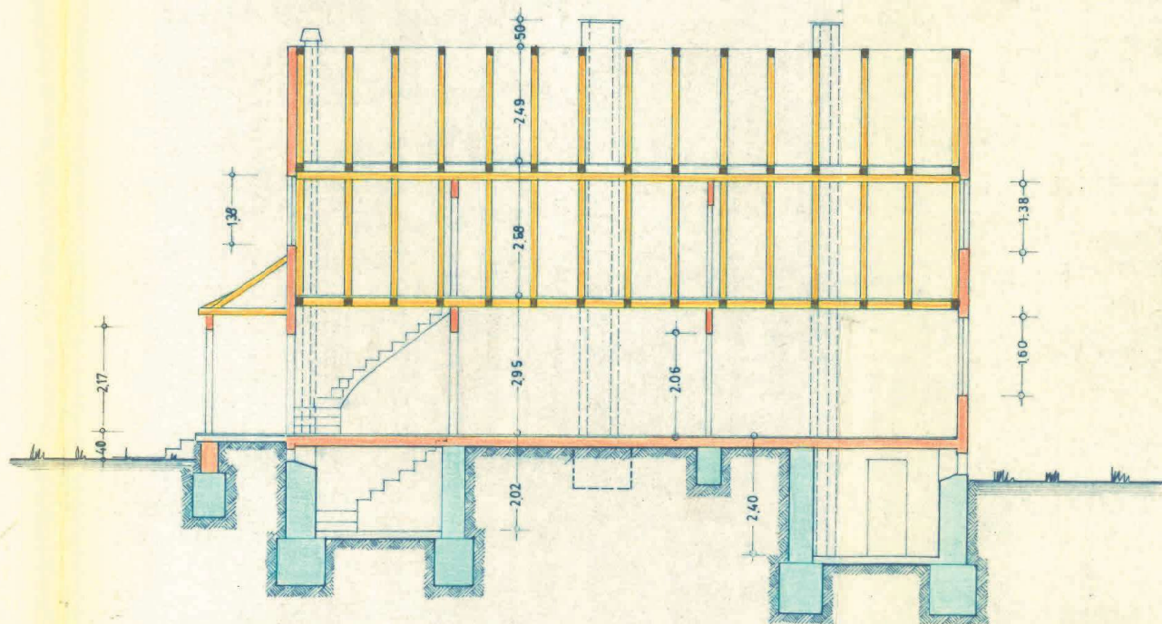
Längsschnitt
