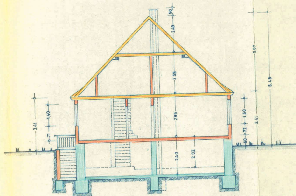
Querschnitt
