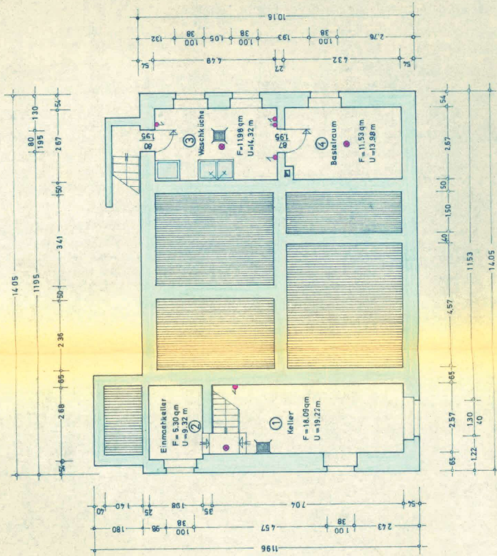
Kellergeschoß
