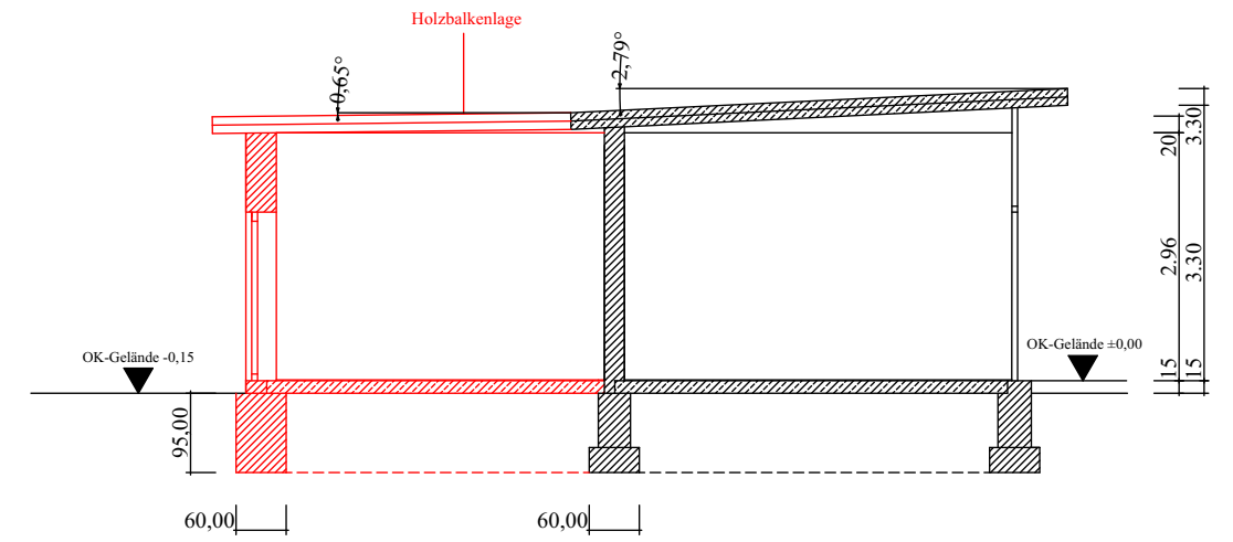
Schnitt B-B
