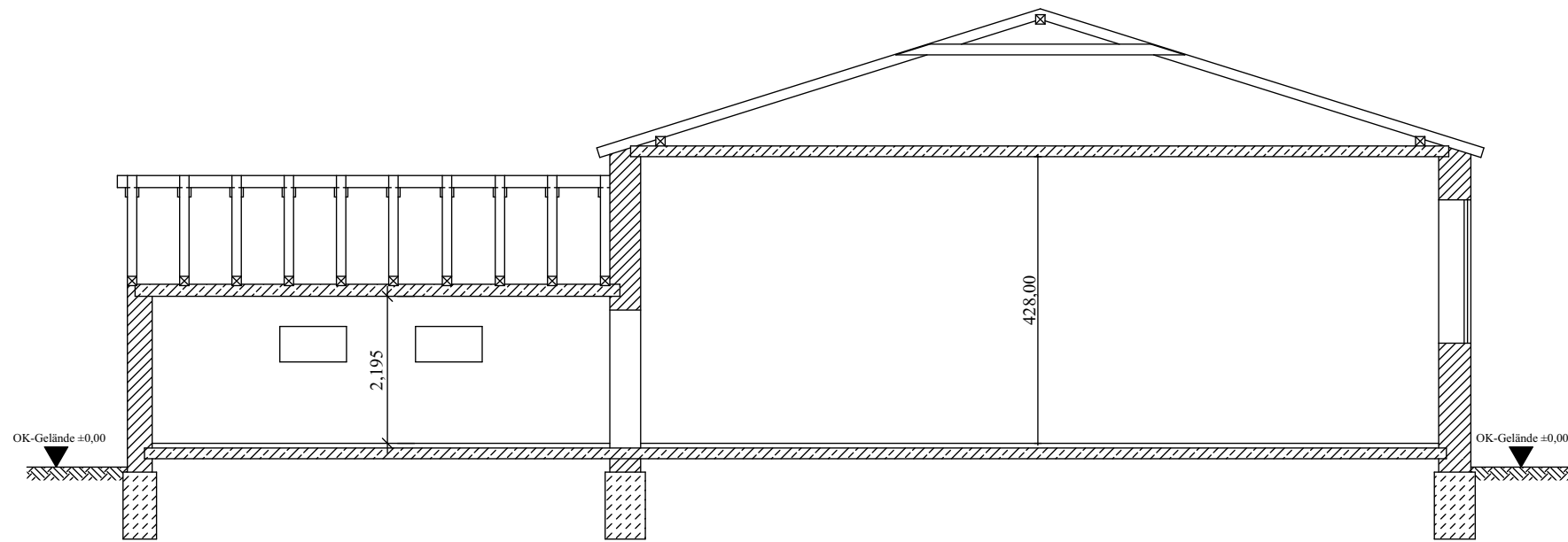
Schnitt A-A
