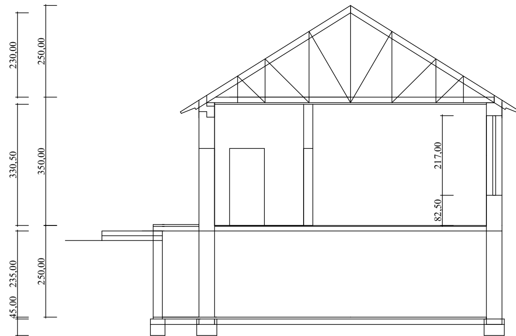
Schnitt Klassentrakt C - C
