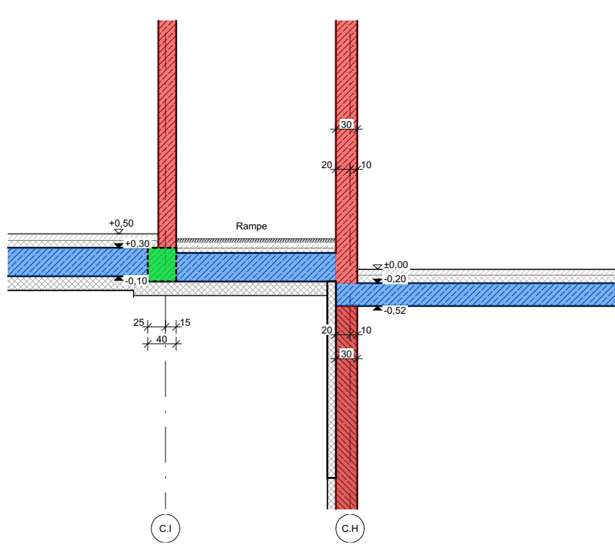
Teilschnitt C.13
