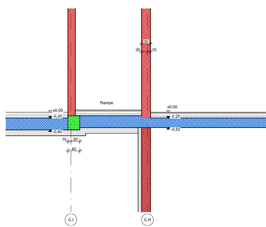
Teilschnitt C.14
