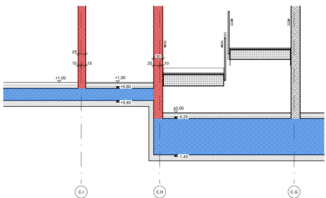
Teilschnitt C.9
