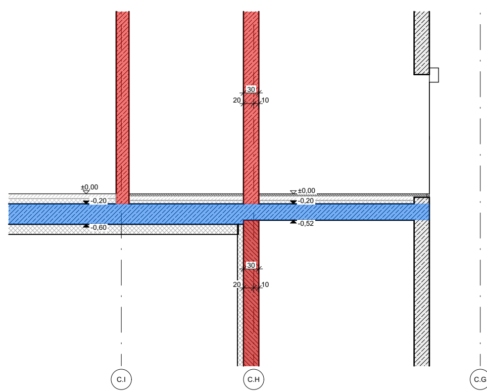
Teilschnitt C.15
