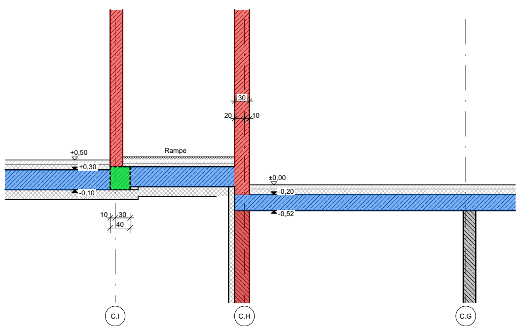
Teilschnitt C.11
