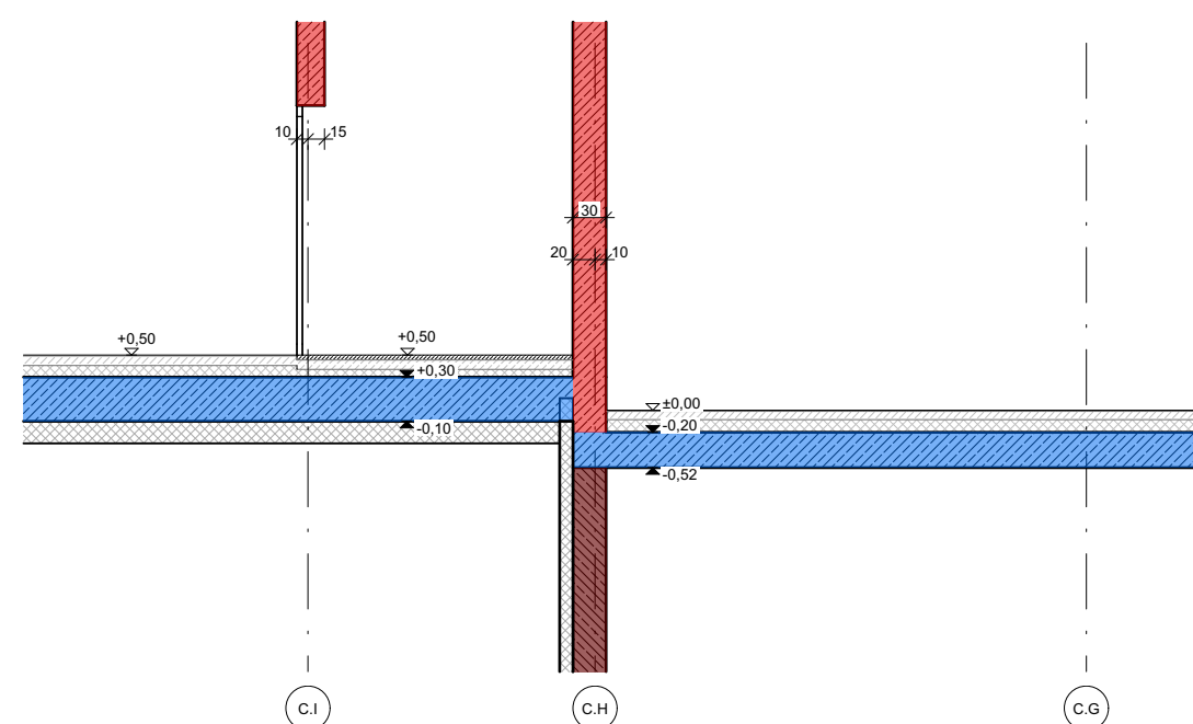
Teilschnitt C.12
