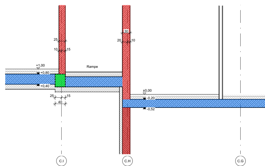
Teilschnitt C.10
