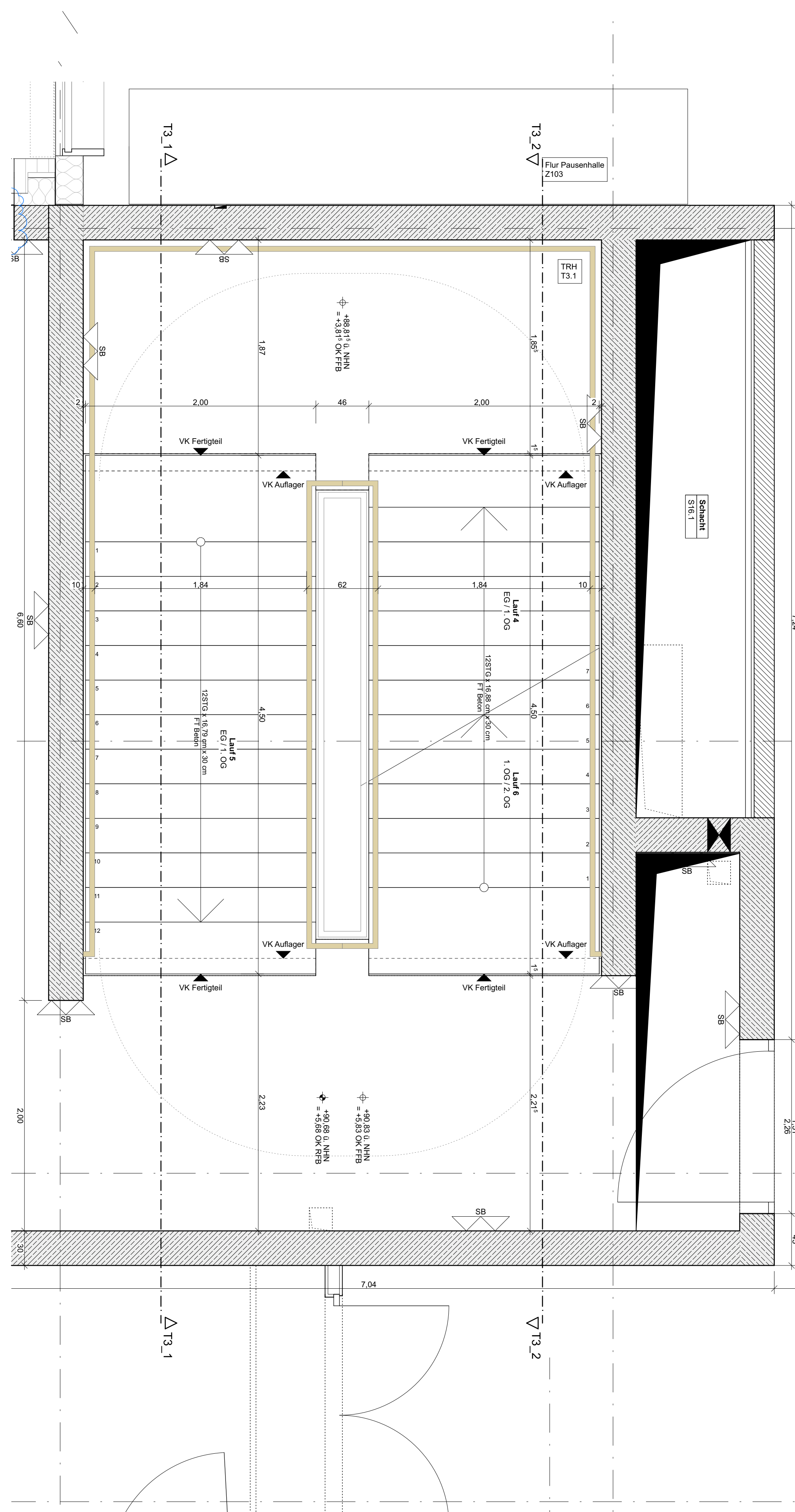
1.Obergeschoss
