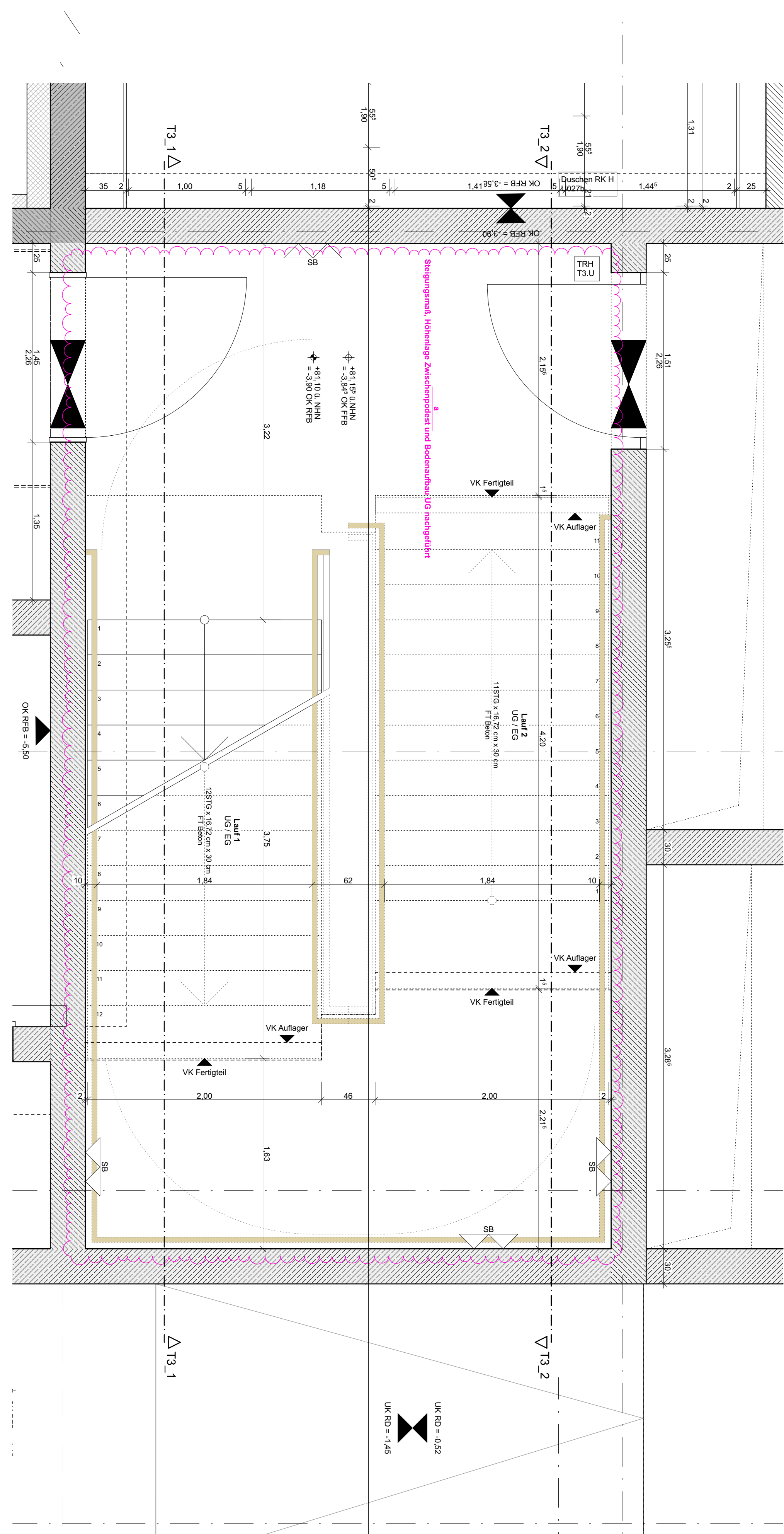
Untergeschoss
