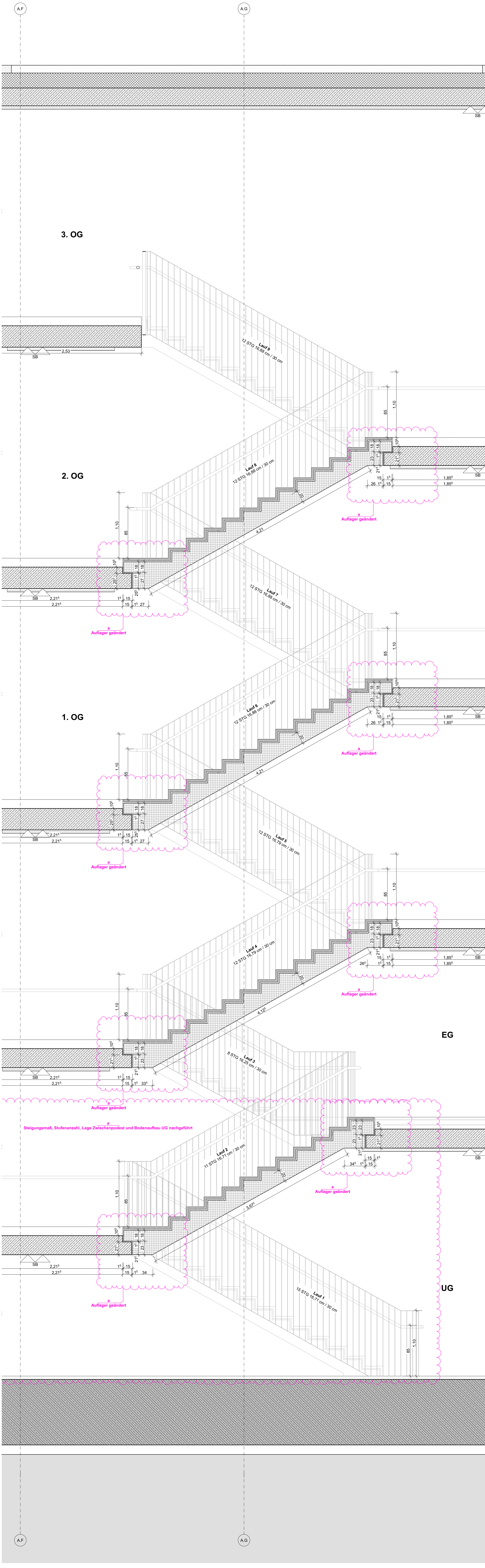
Schnitt T1_2
