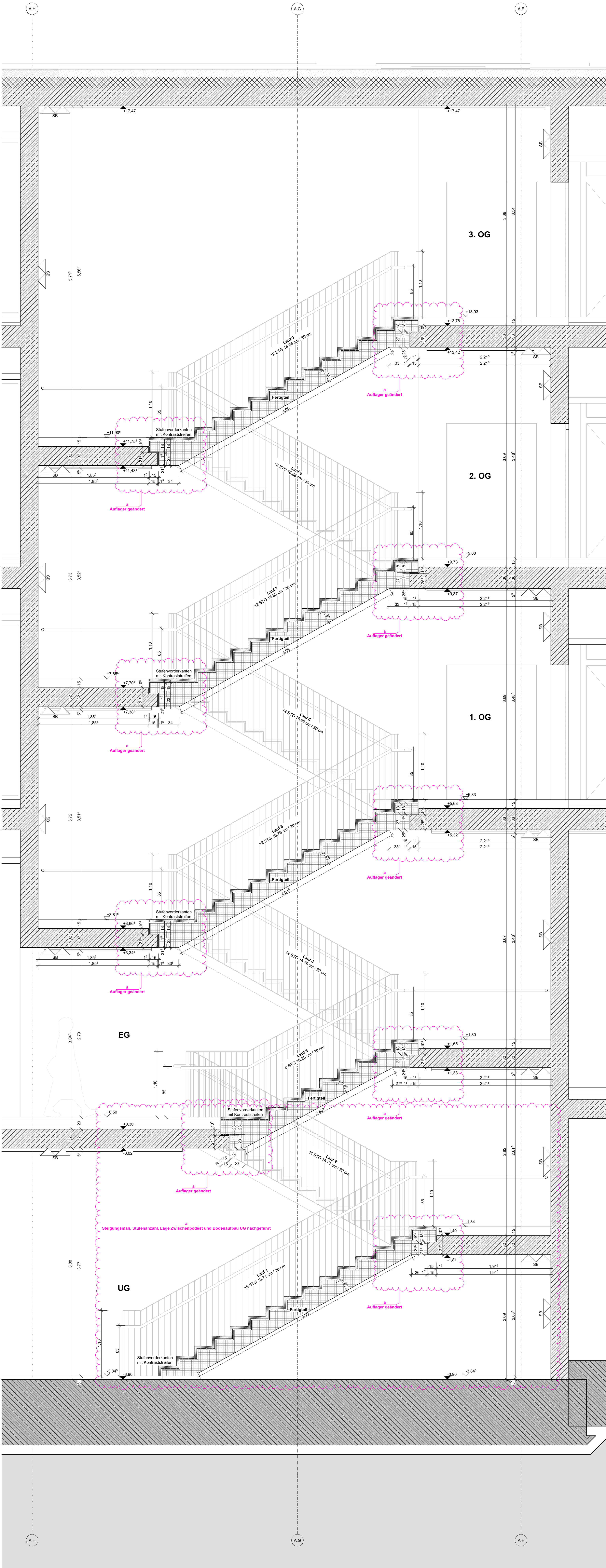
Schnitt T1_1
