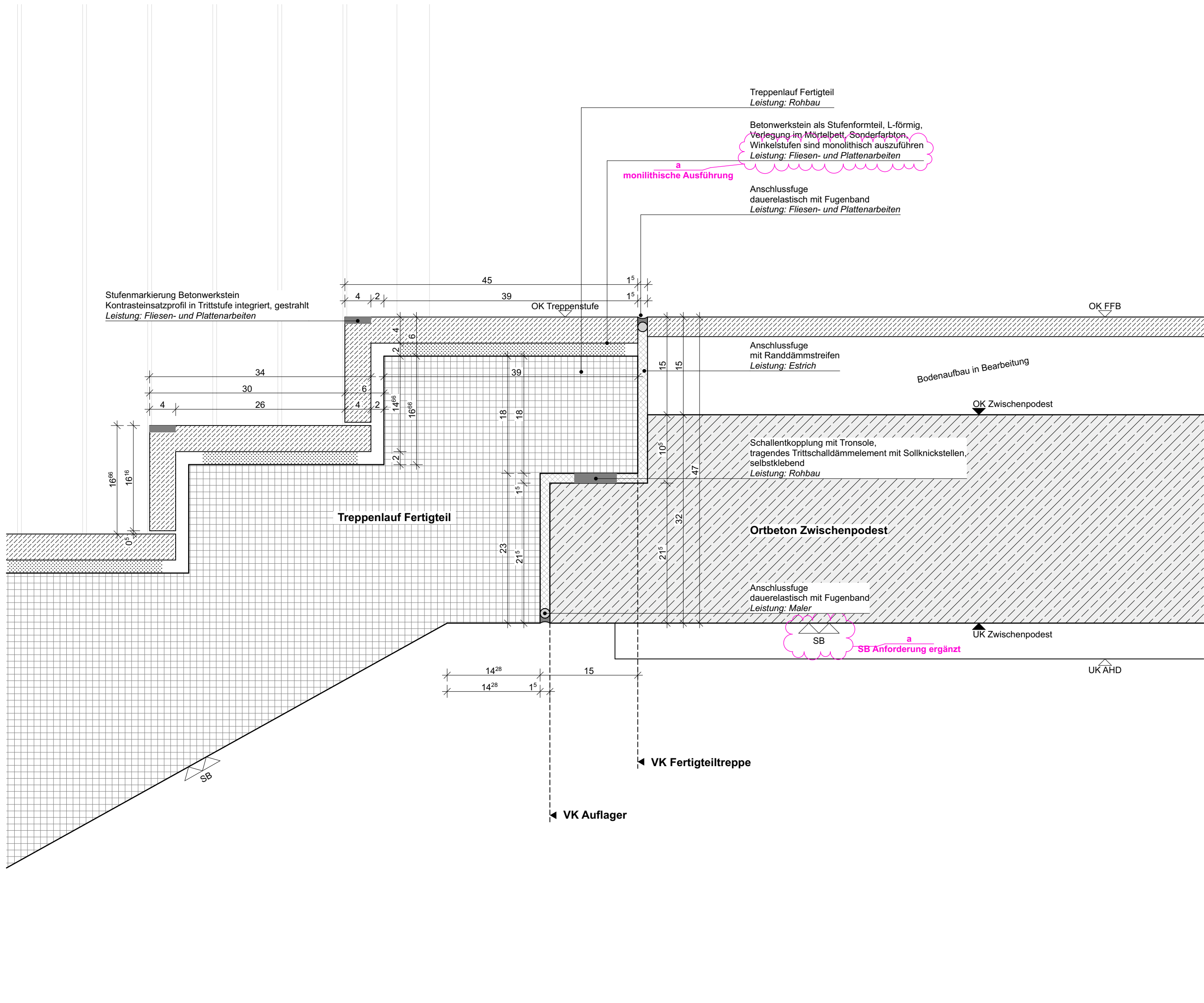
DE04 Regeldetail Anschluss FT-Lauf an Zwischenpodest - 18cm Auflager
