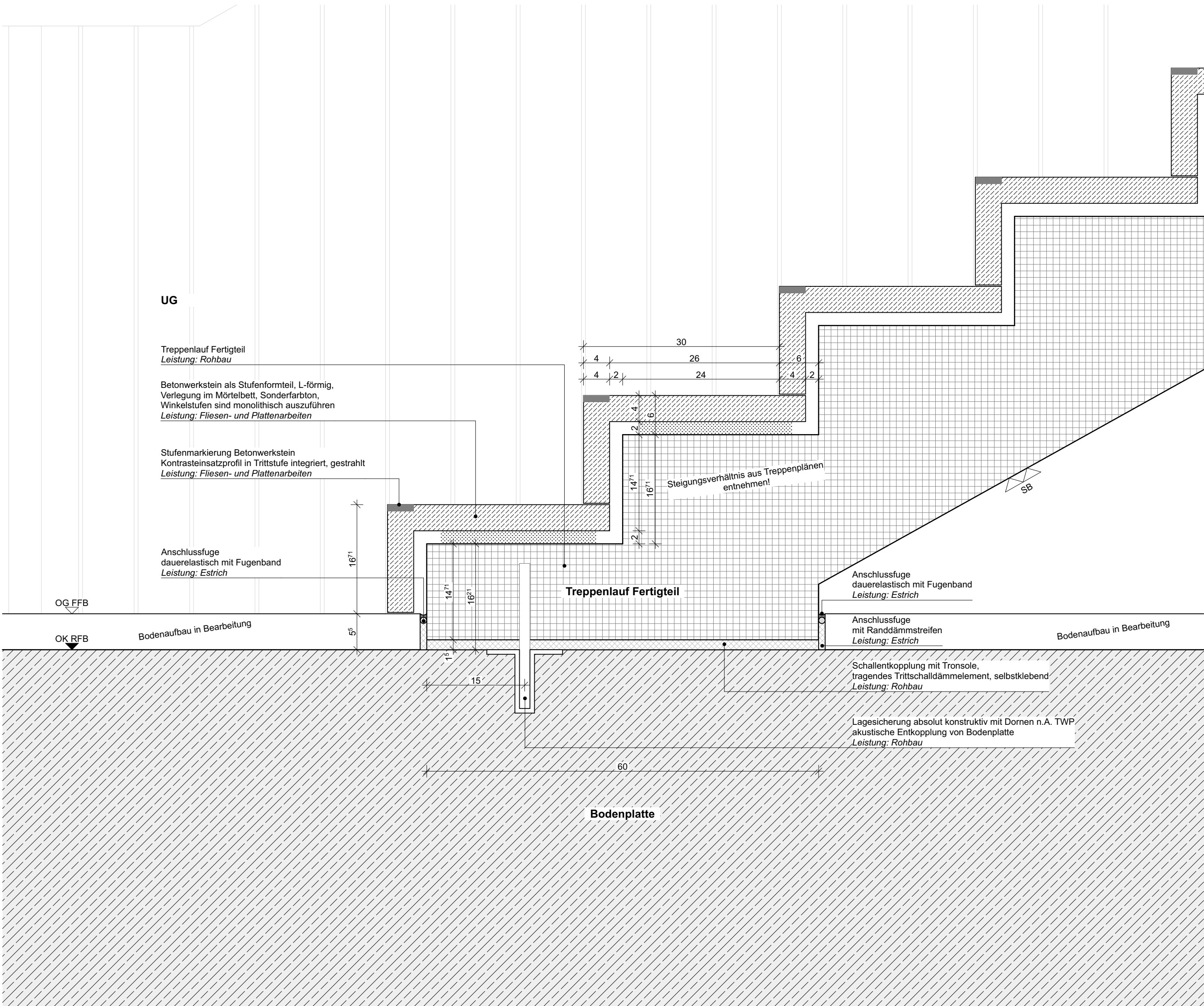
DE02 Regeldetail Treppenaufleger an UG STB-Bodenplatte
