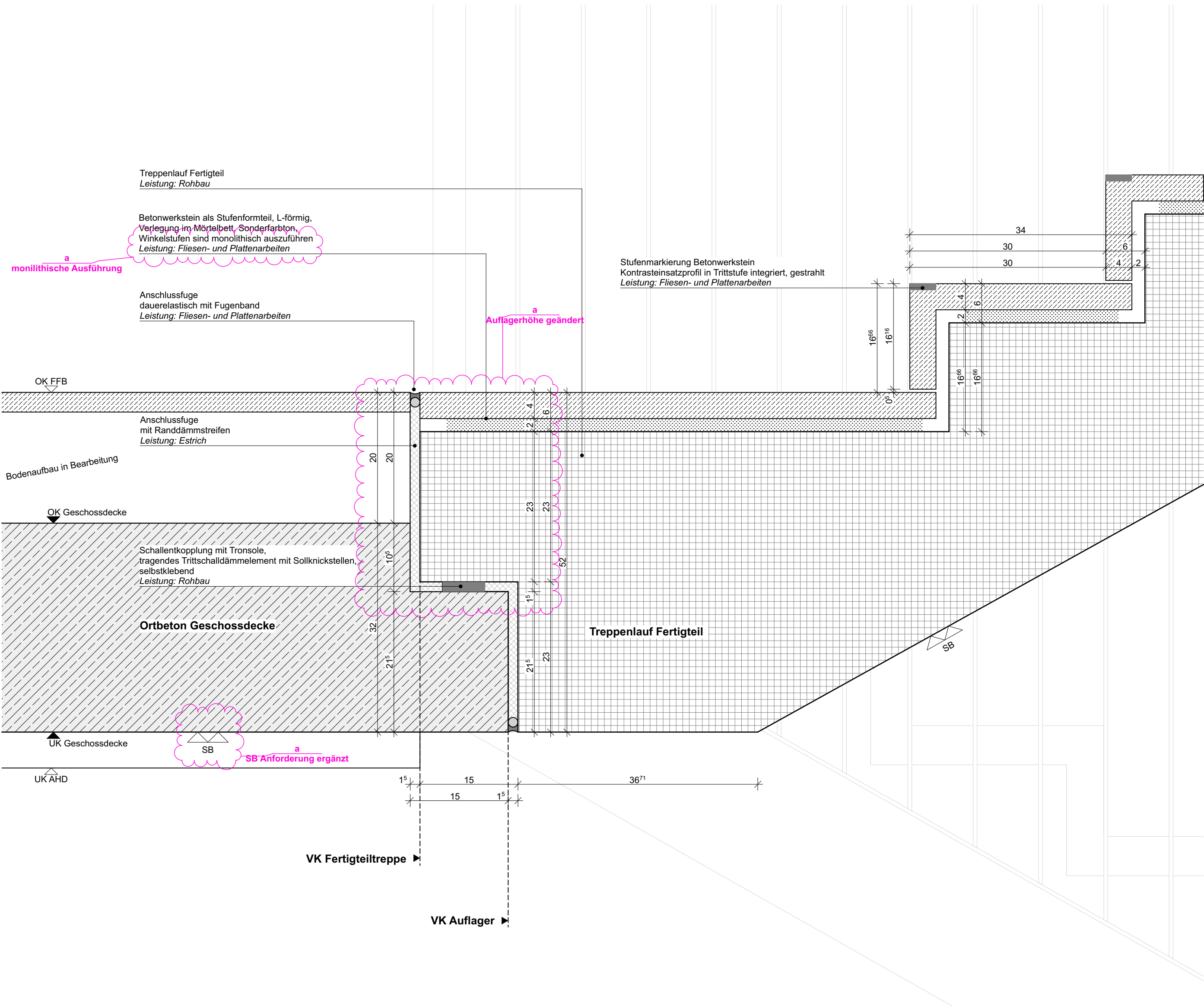
DE03 Regeldetail Anschluss FT-Lauf an EG Geschosdecke - 23cm Auflager
