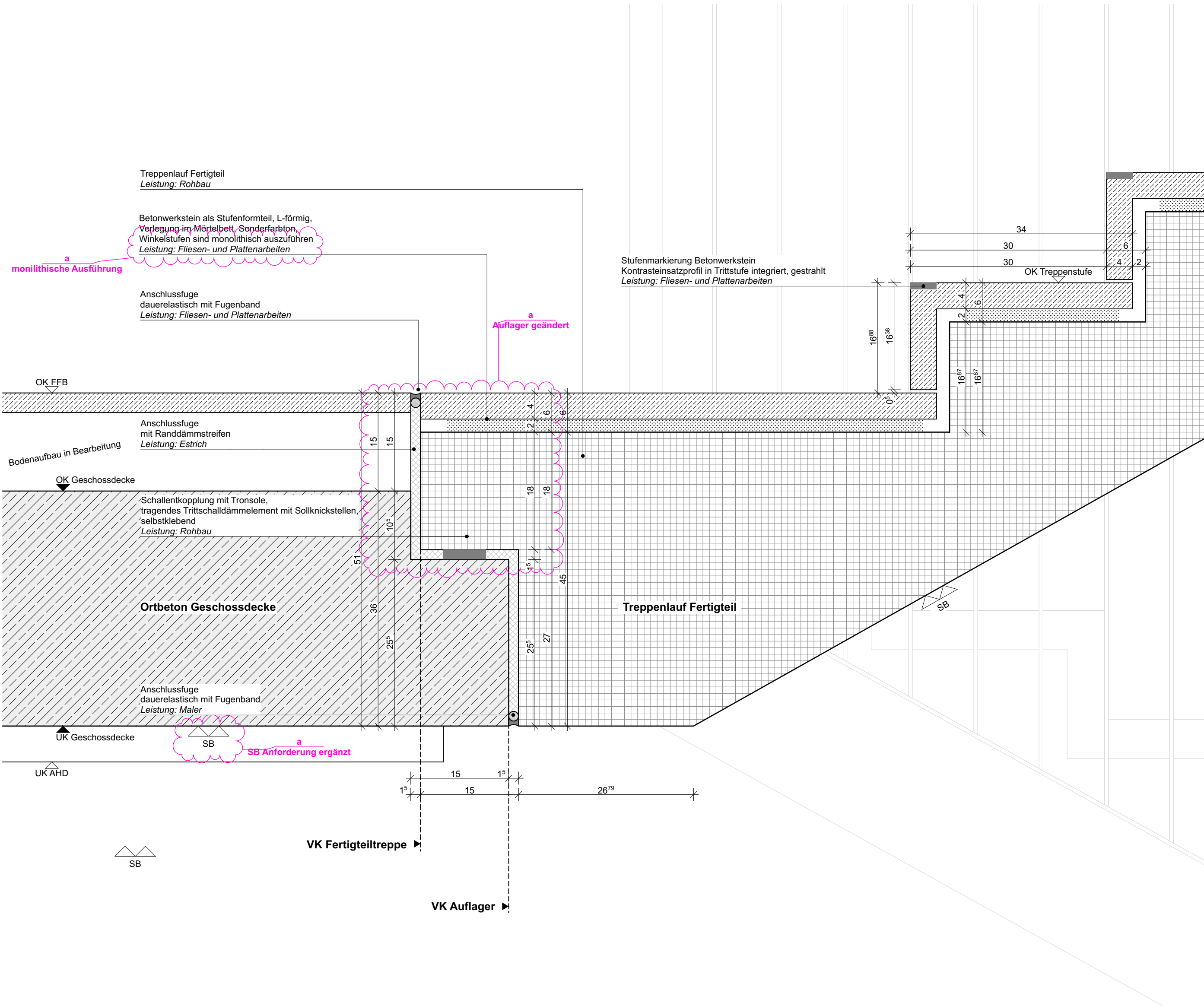
DE05 Regeldetail Anschluss FT-Lauf an Geschosdecke - 18cm Auflager
