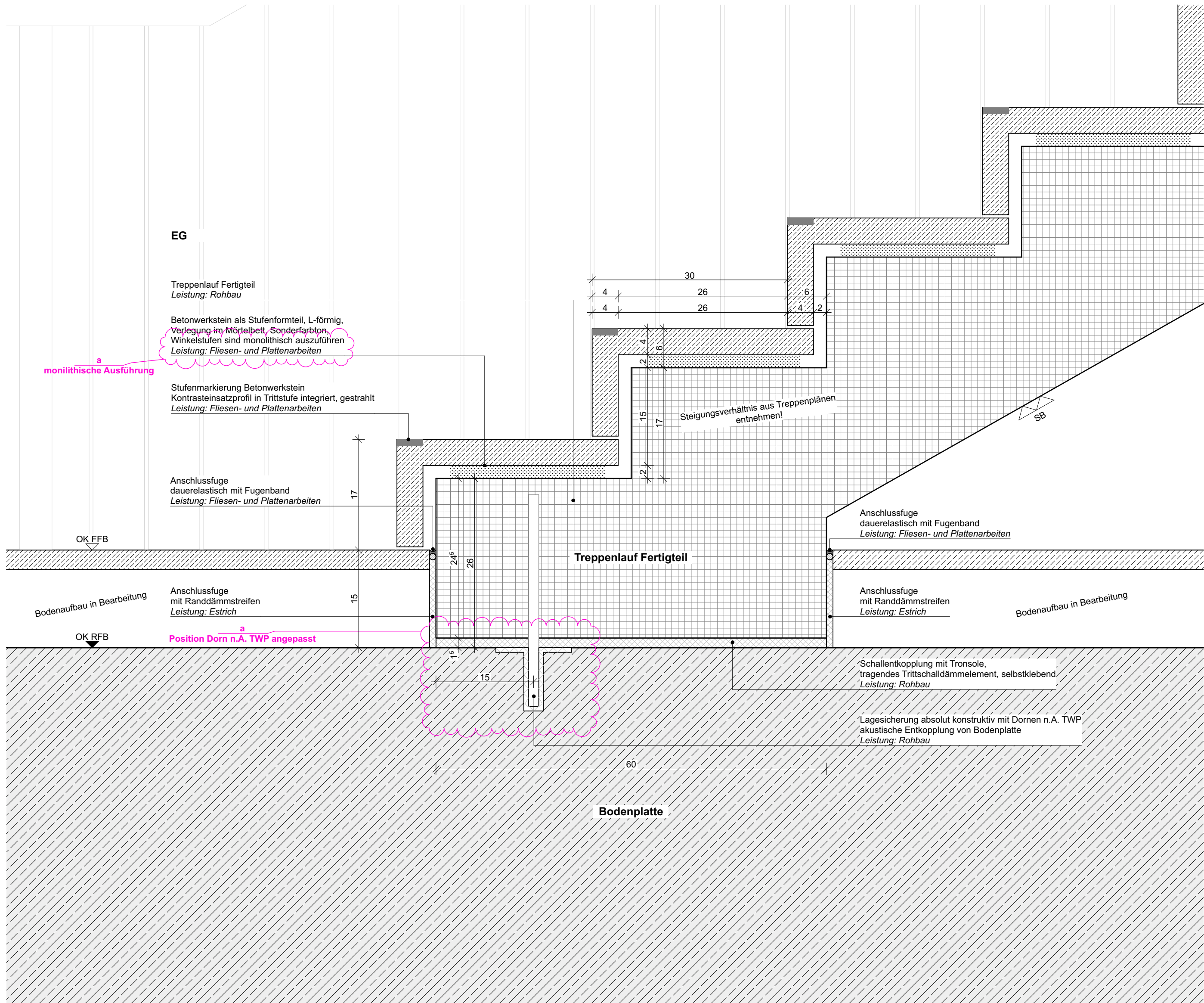
DE01 Regeldetail Treppenaufleger an EG STB-Bodenplatte
