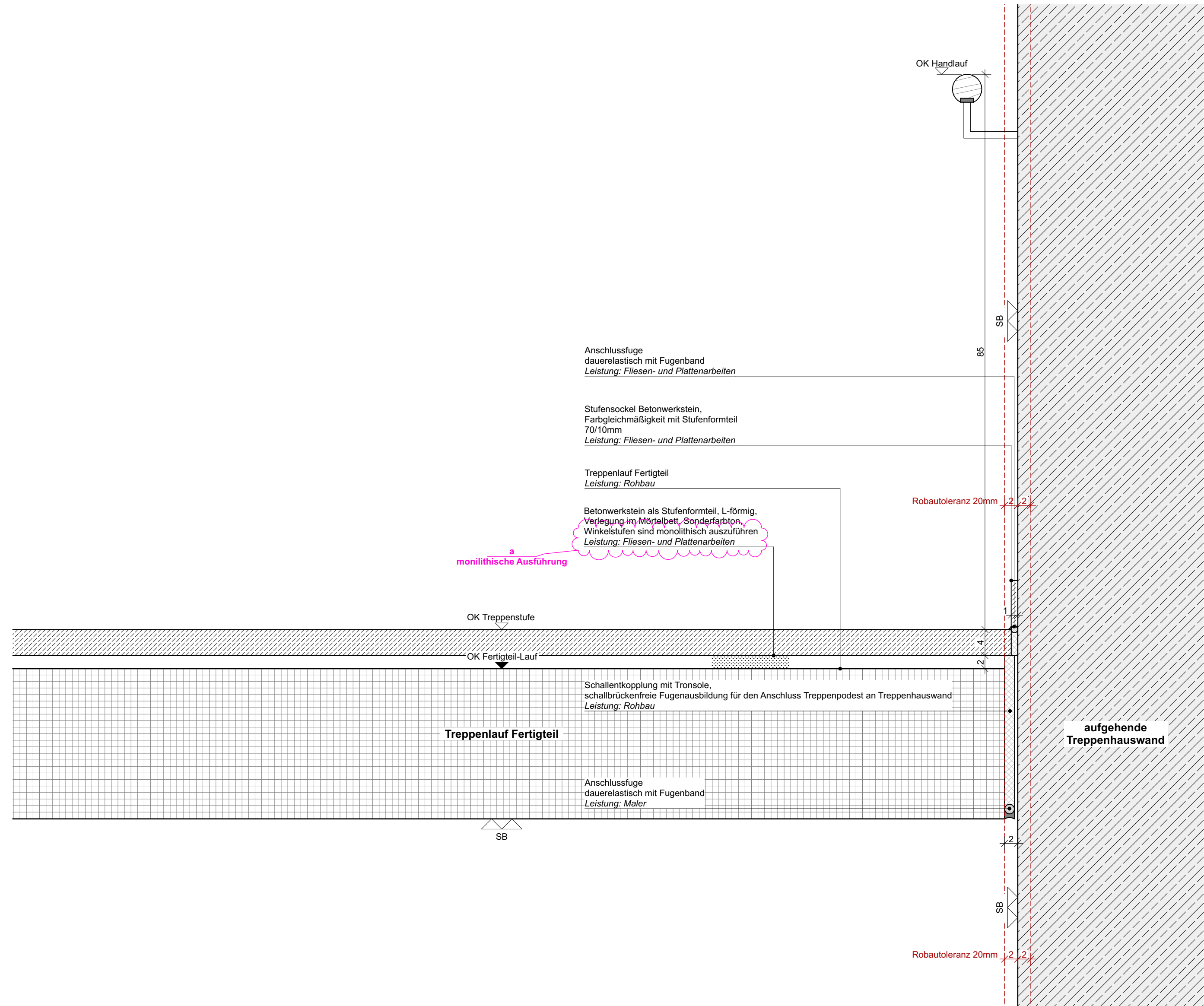
DE06 Detail Anschluss Fertigteilauflauf an aufgehende Wand
