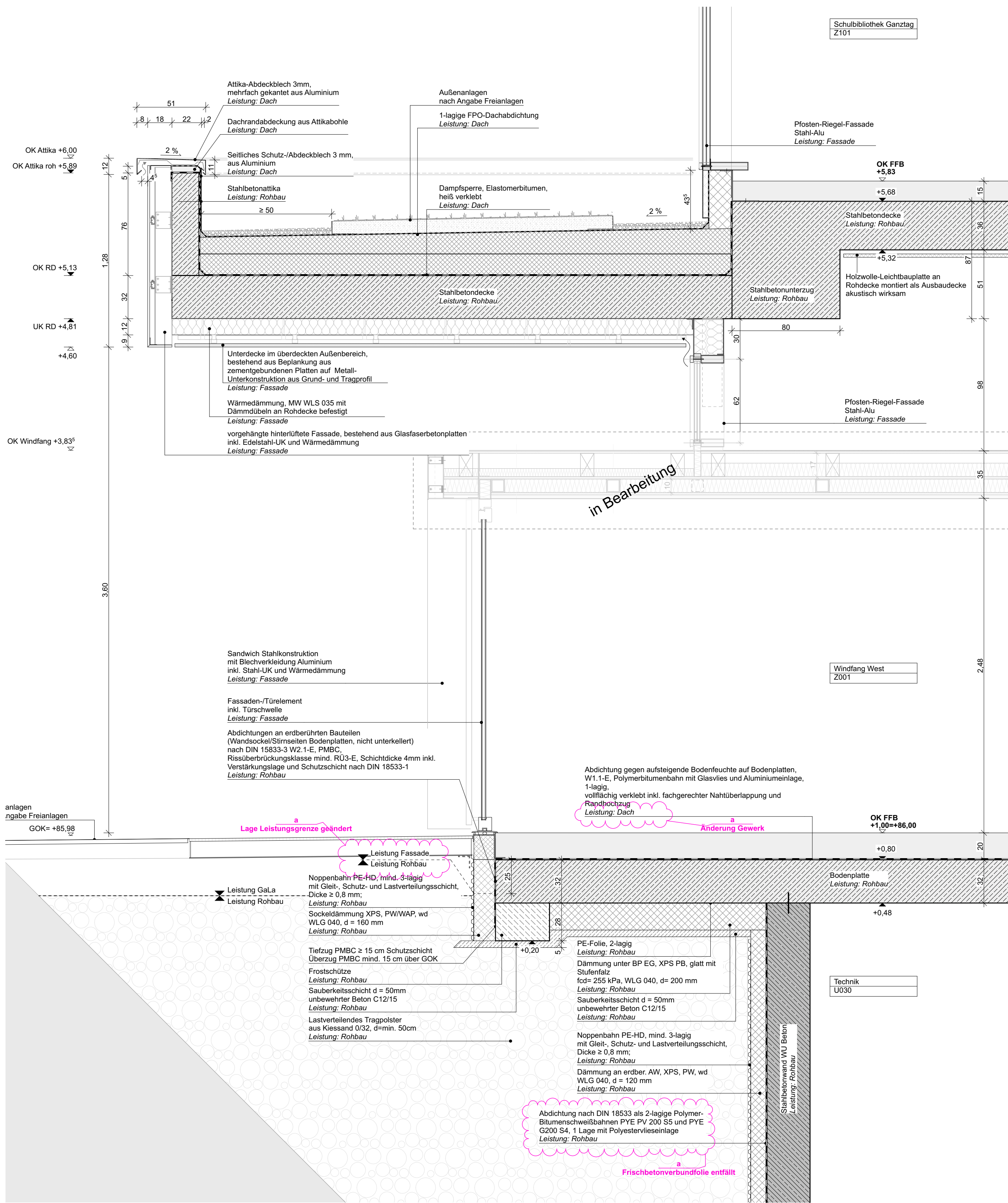
DE01 Windfang West Bereich Vordach und Bodeplatte auf Frostschiene und erdbAußenwand M1:20
