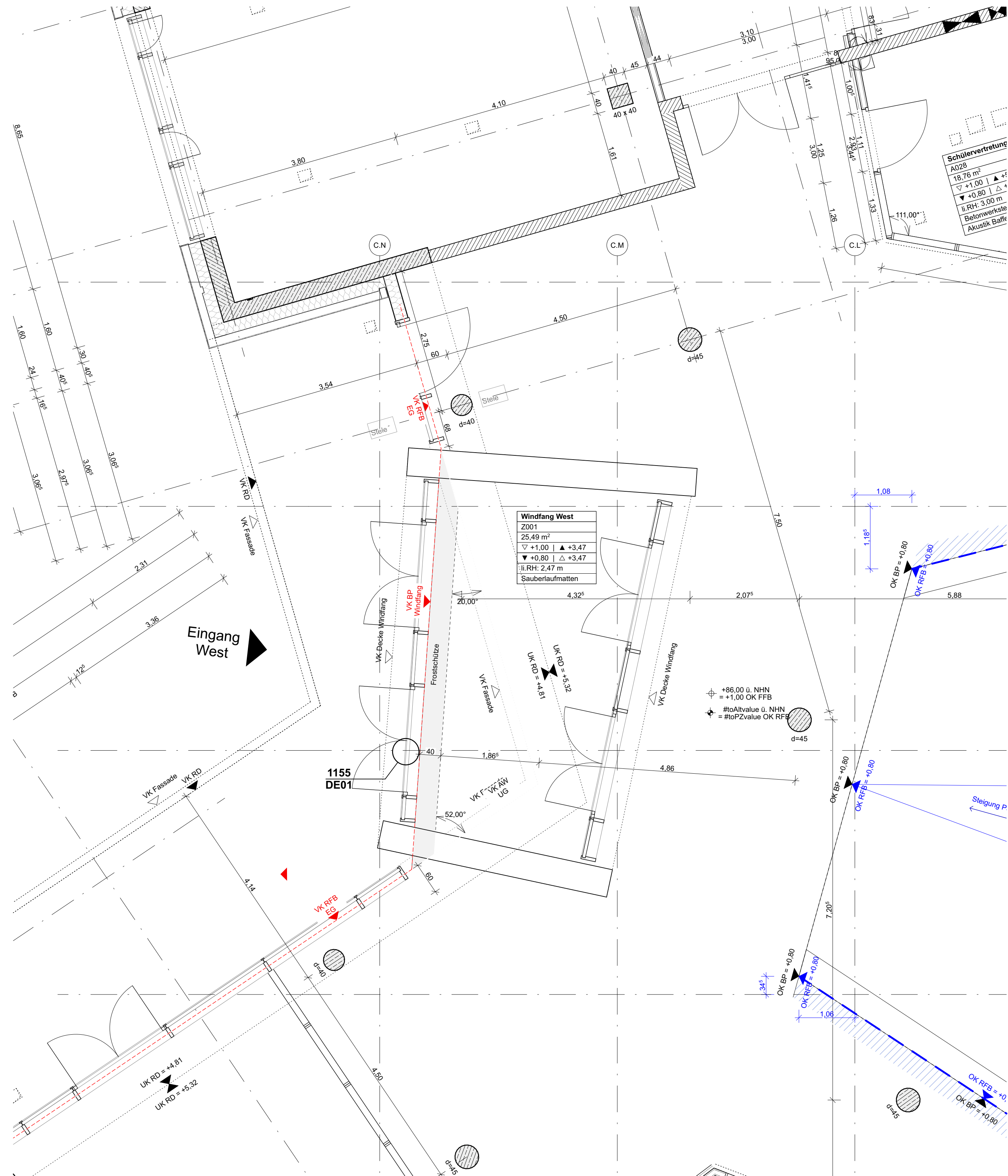
EG Grundriss Ausschnitt Windfang West M1:50
