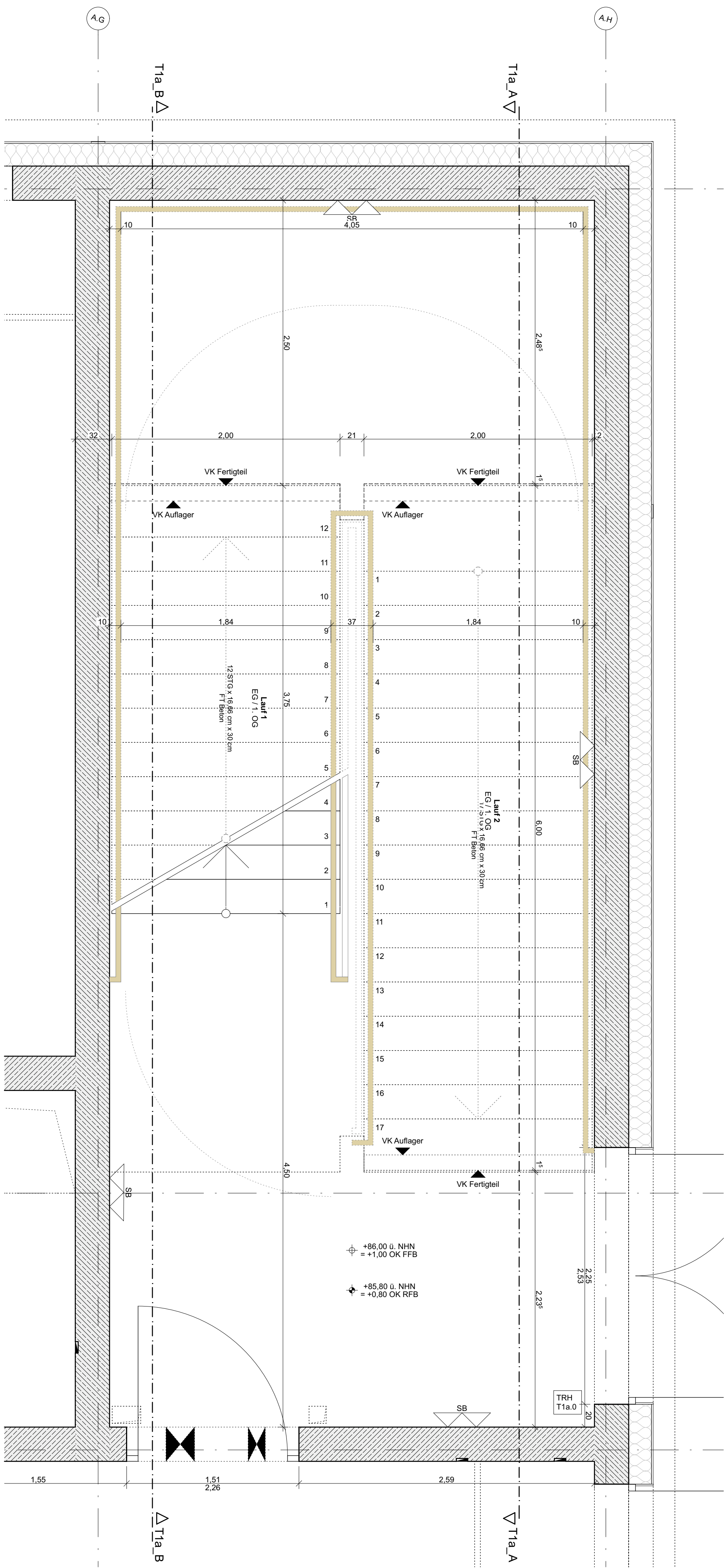
Erdgeschoss
