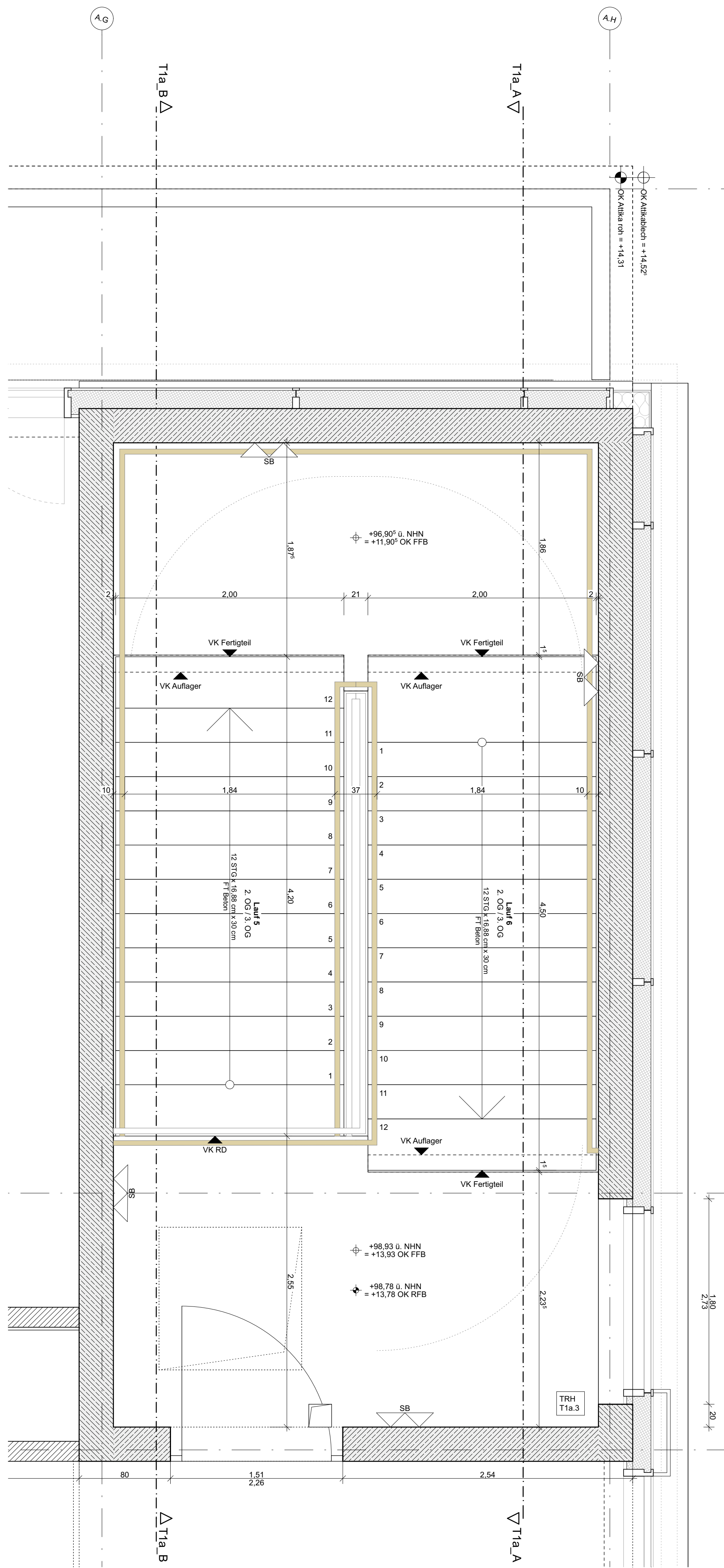
3.Obergeschoss
