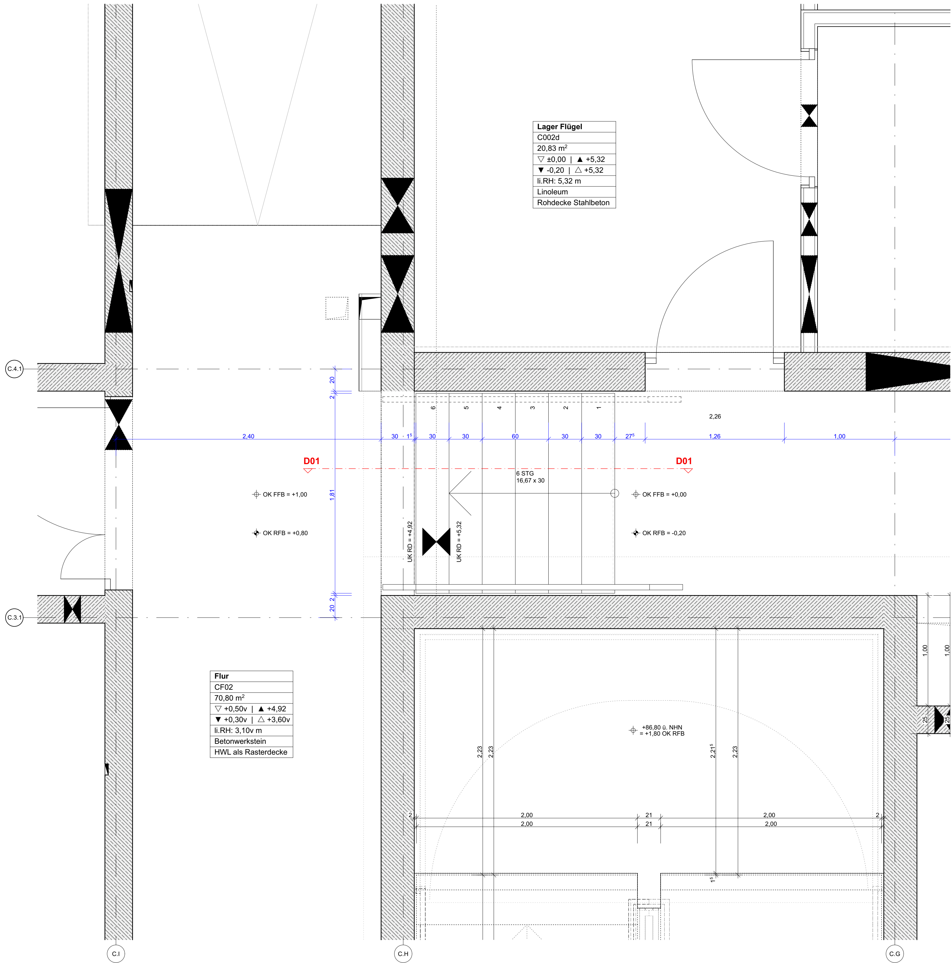
Grundriss Stufenanlage BT C - Übergang Aula zu Flur Zwischenbau
