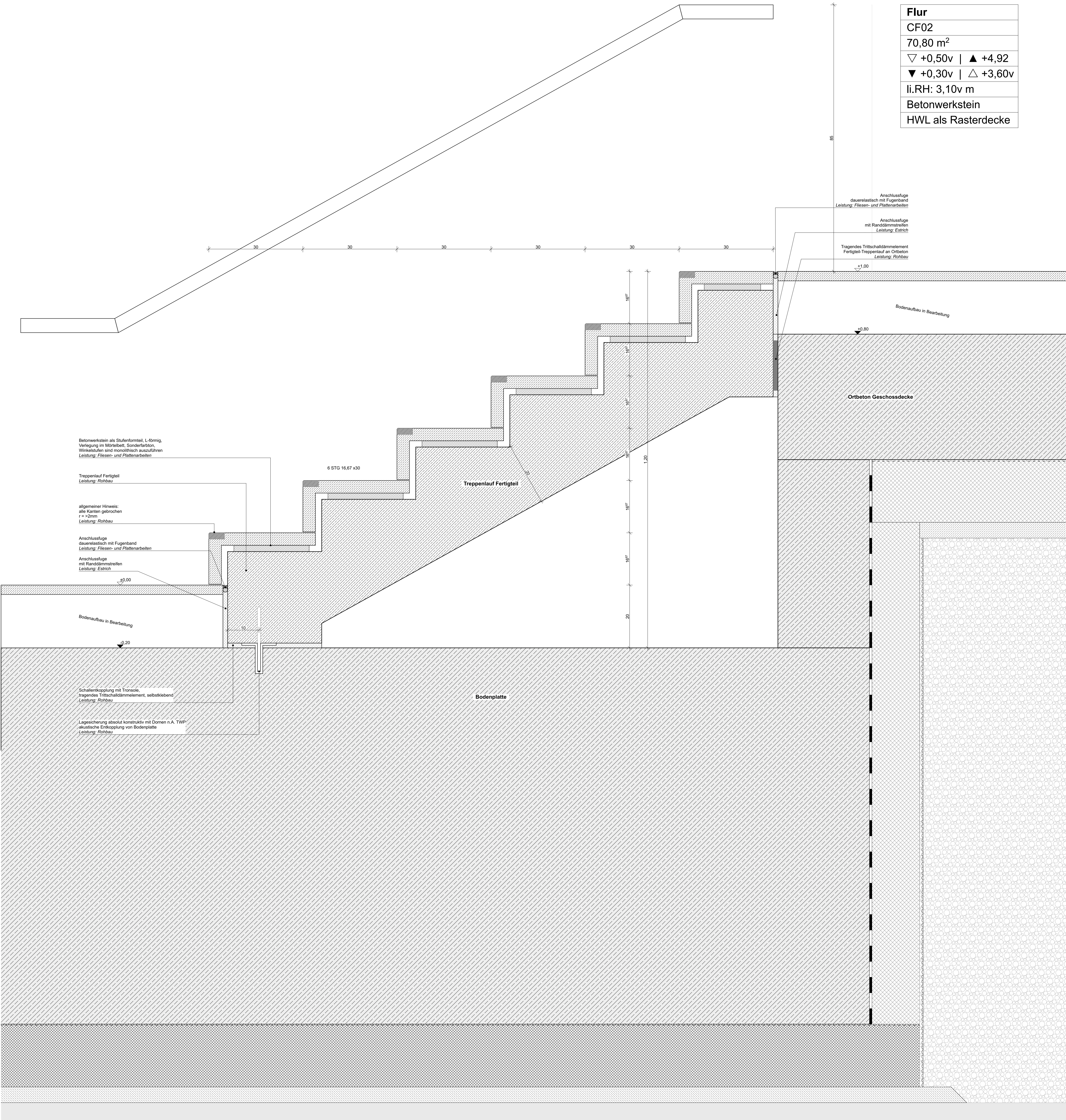
DE01 Regeldetail FT-Treppe mit Betonwerkstein
