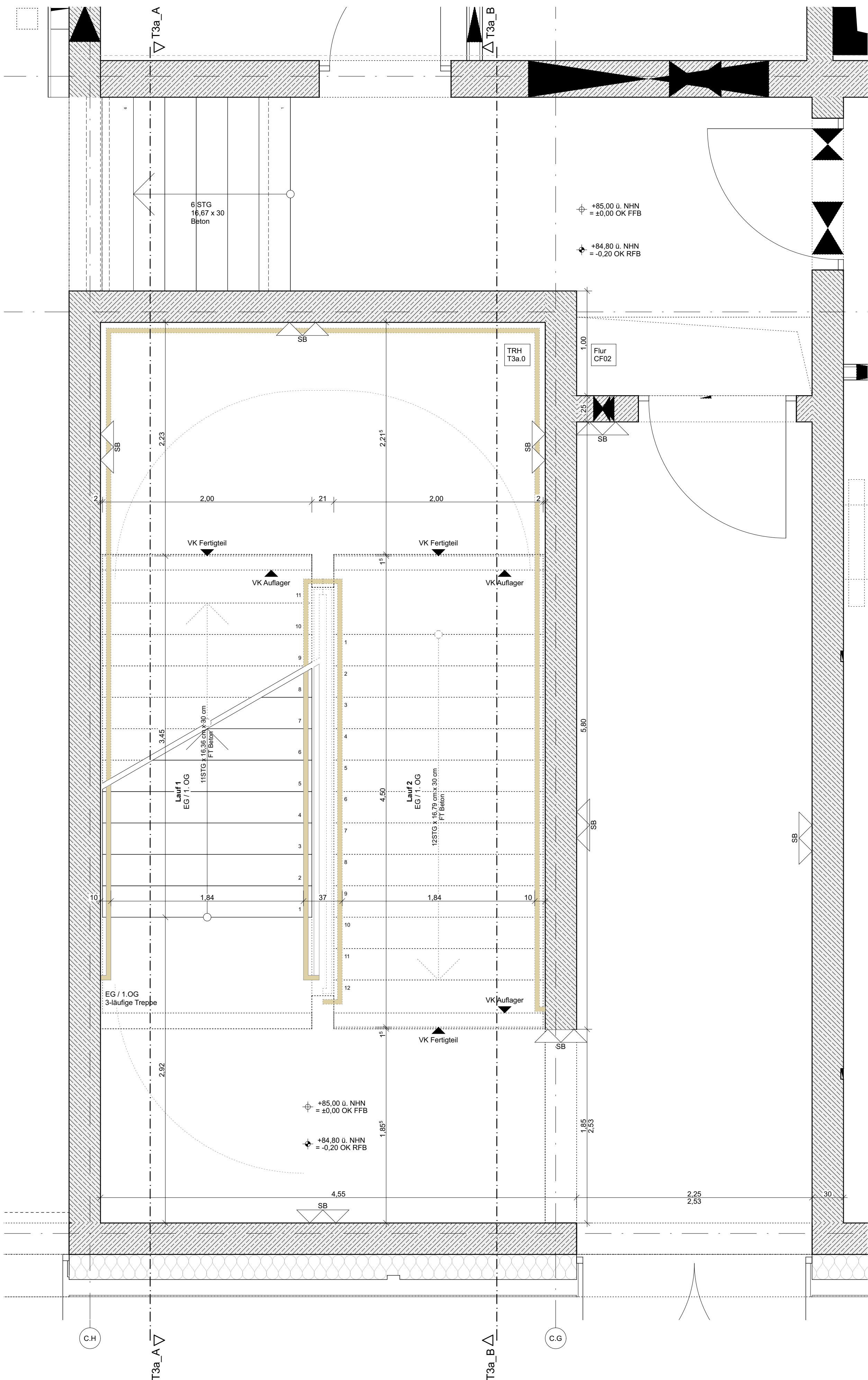
Erdgeschoss
