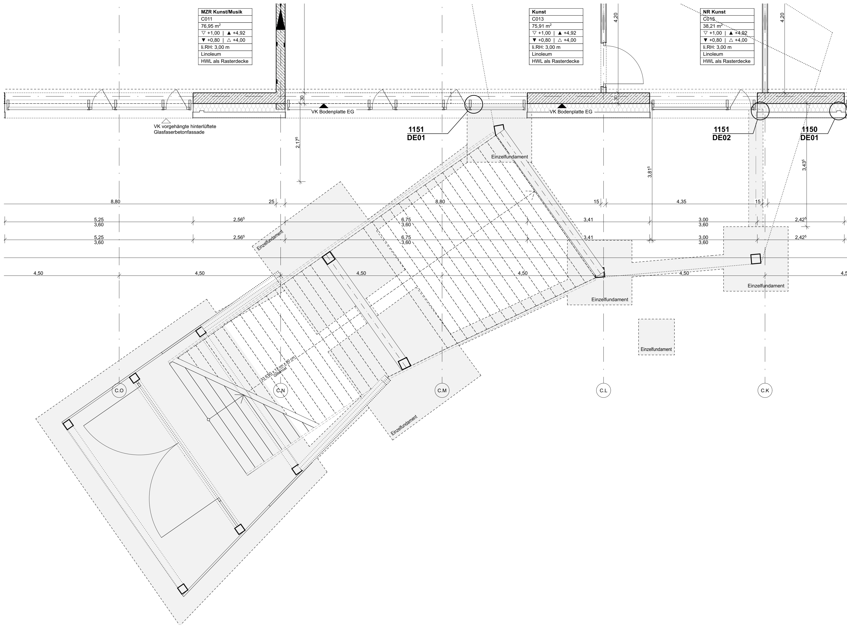
EG Grundriss Ausschnitt M1:50
