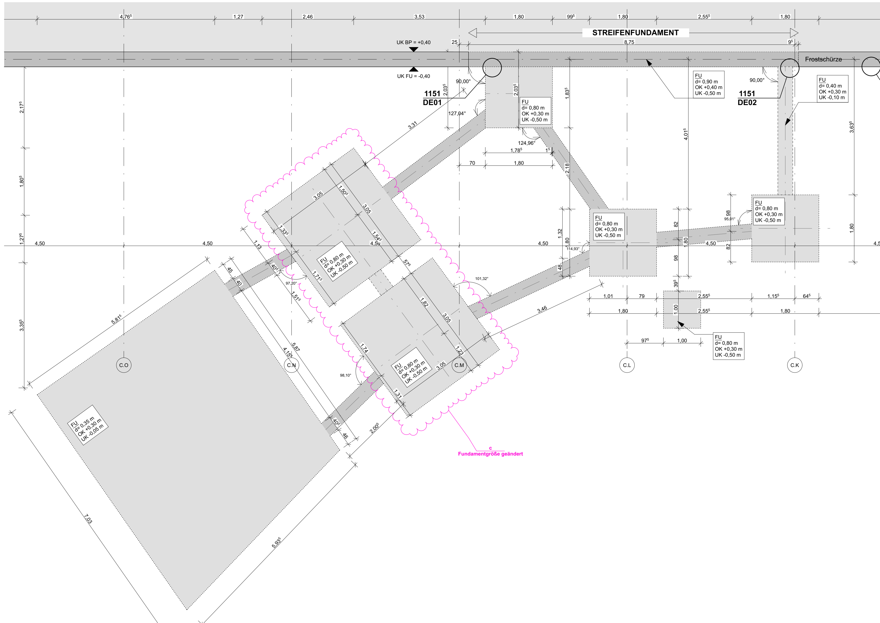
Fundamentenplan Ausschnitt M1:50
