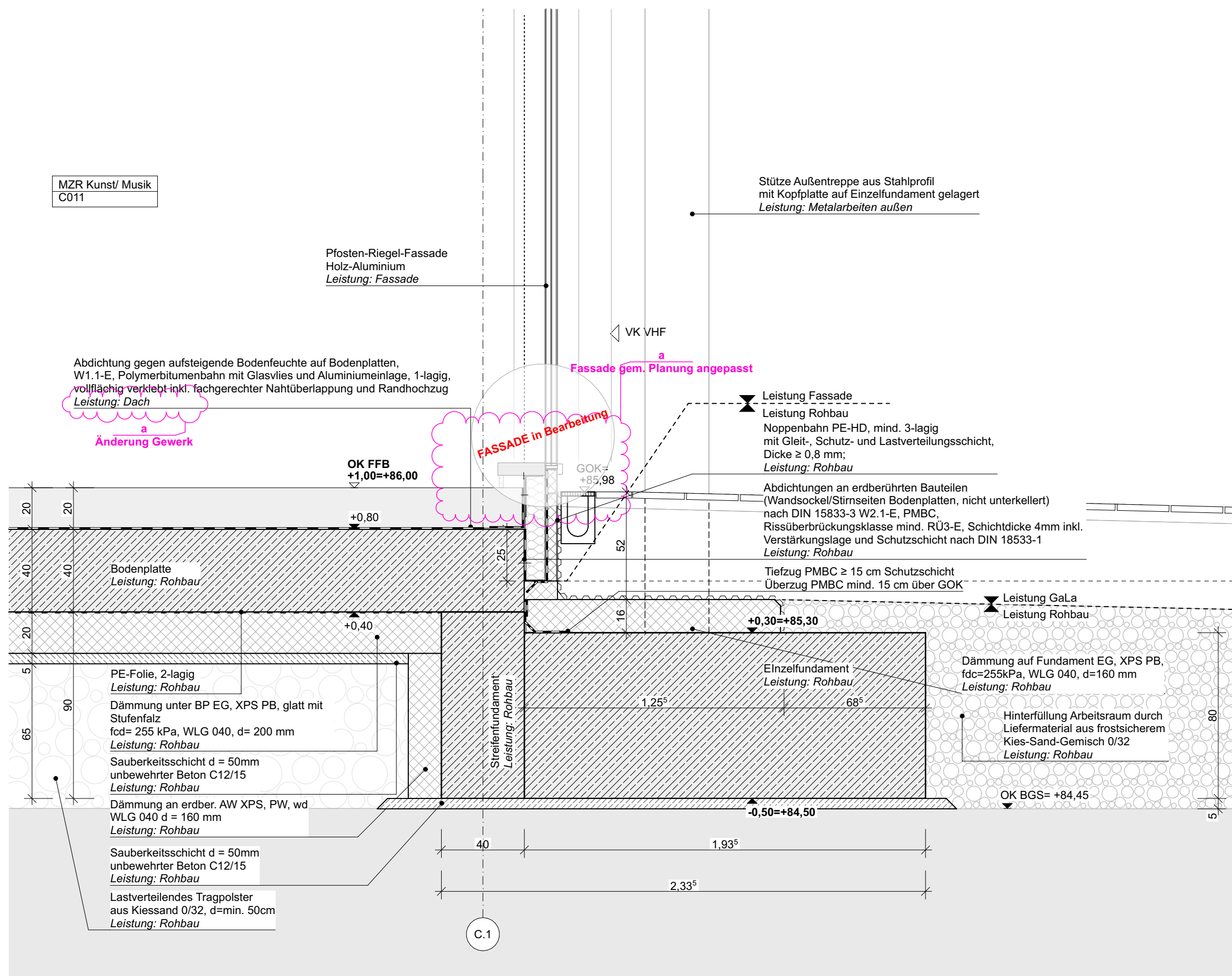
DE01 Bodenplatte EG Bauteil C Bereich Zwischenbau Außen-/Fluchttreppe mit Streifen- und Einzelfundament / Außenwand mit VHF
