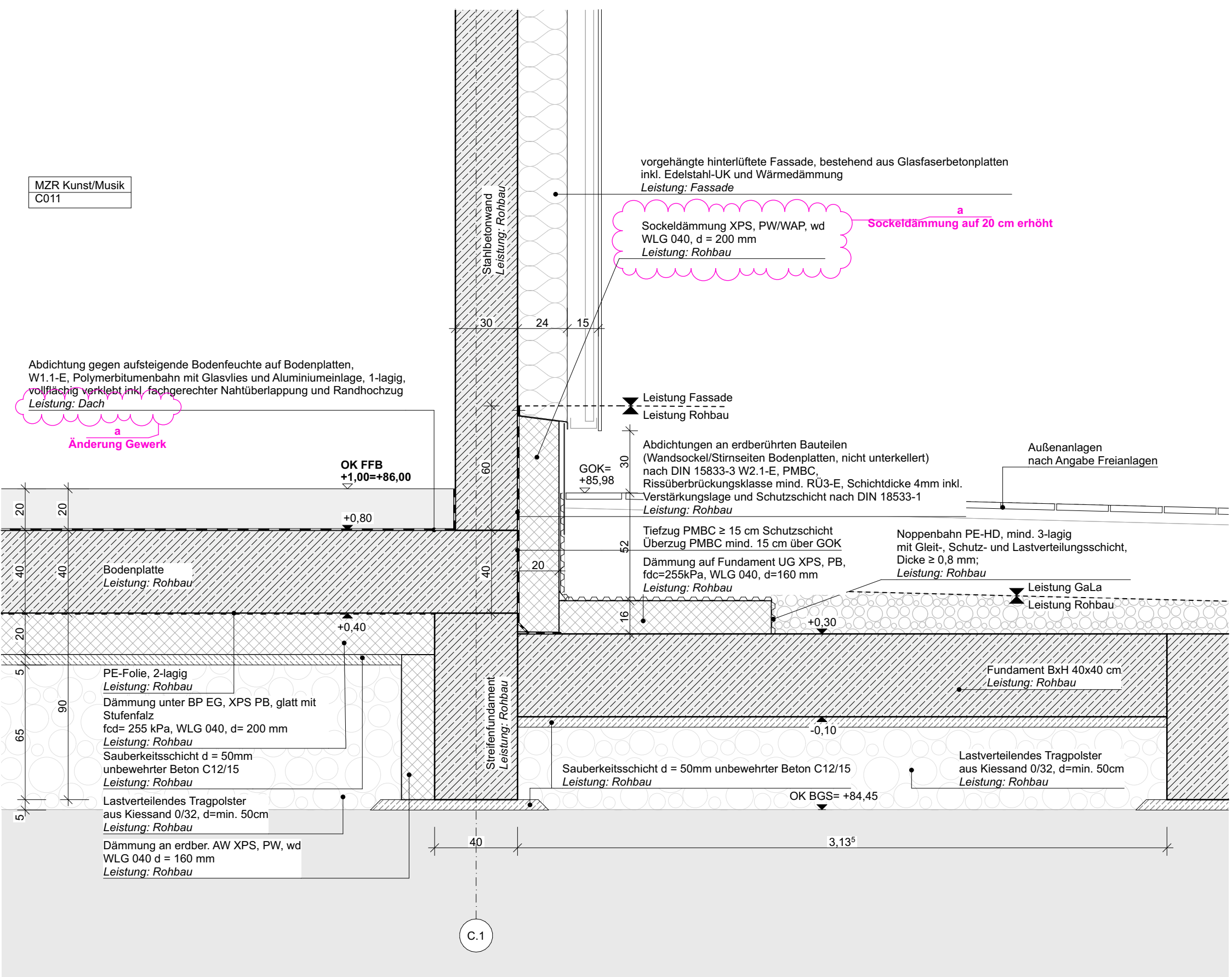
DE02 Bodenplatte EG Bauteil C Bereich Zwischenbau Außen-/Fluchttreppe mit Streifenfundament/ Zerrbalken / Außenwand mit VHF
