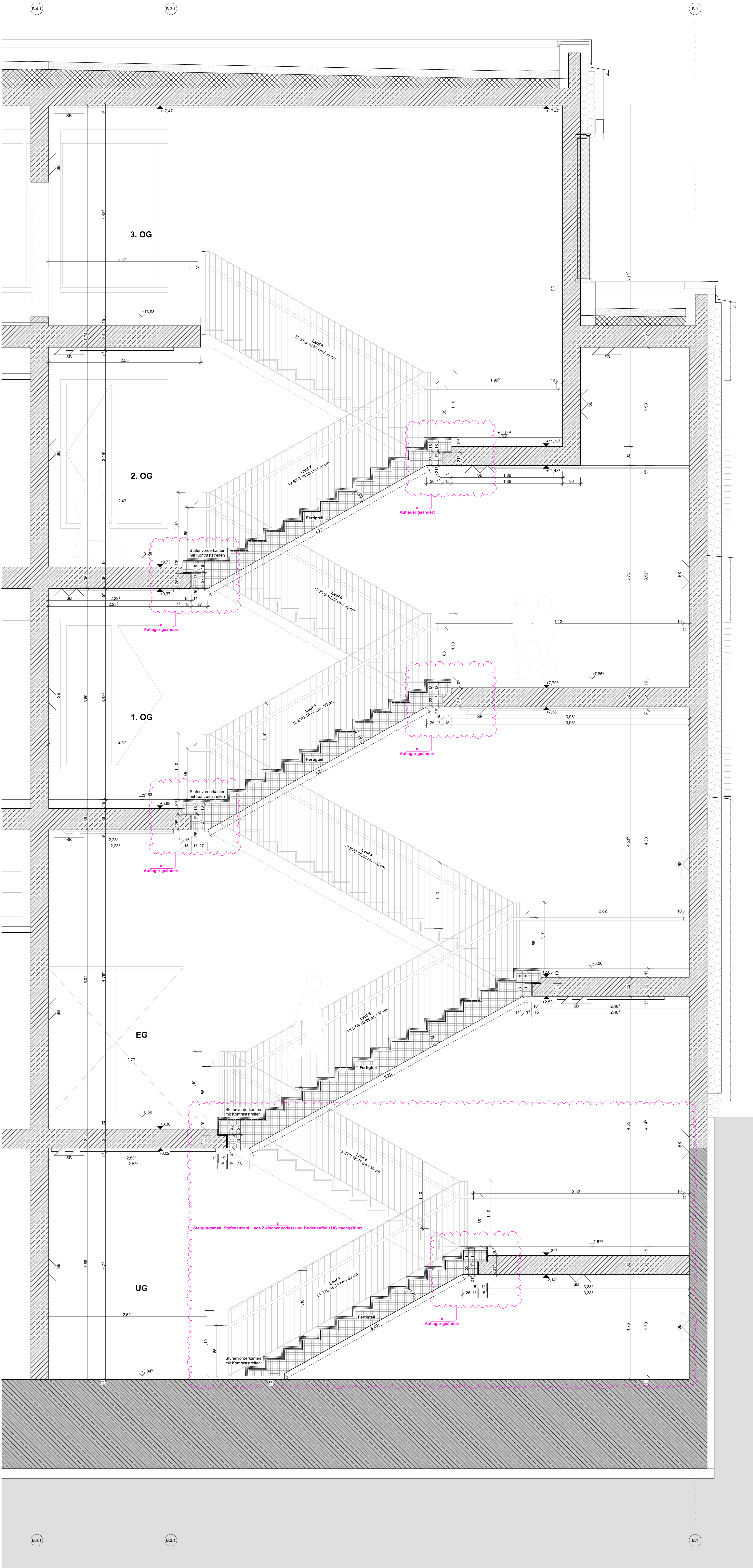
Schnitt T2a_B
