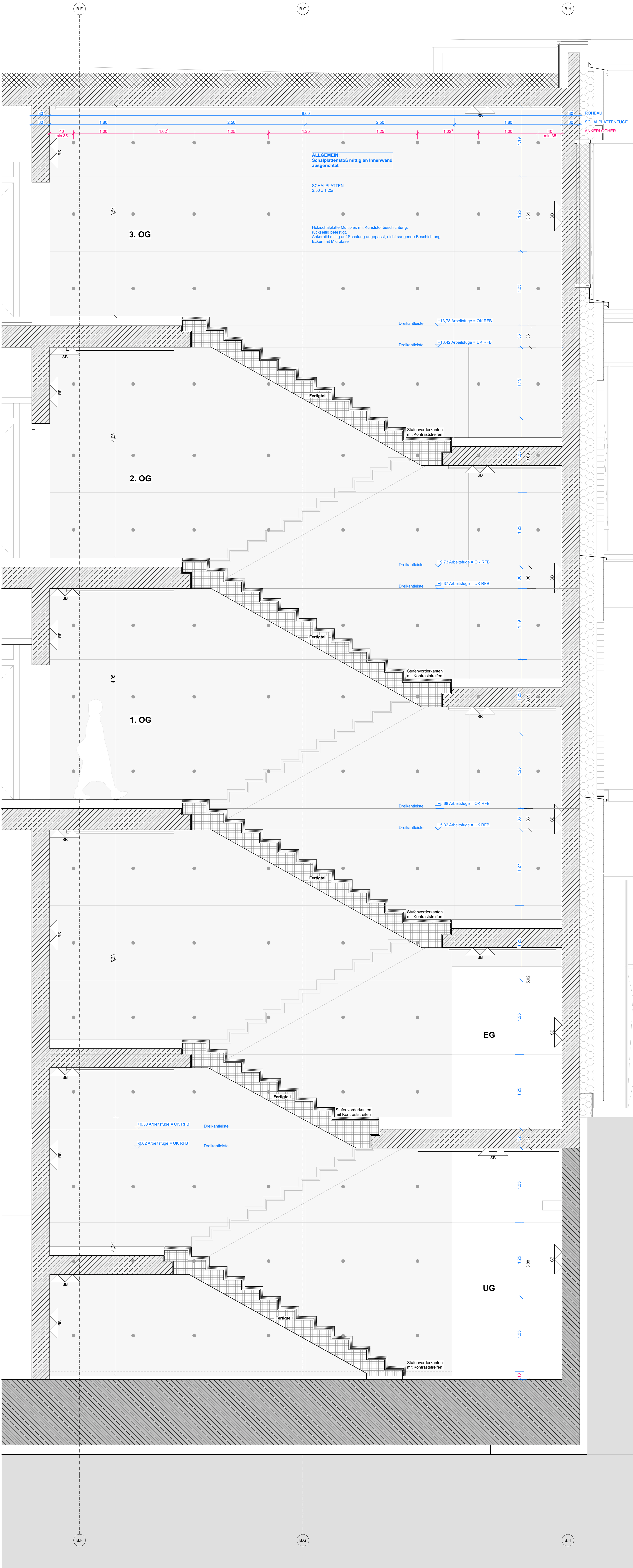
Schnitt T2_1
