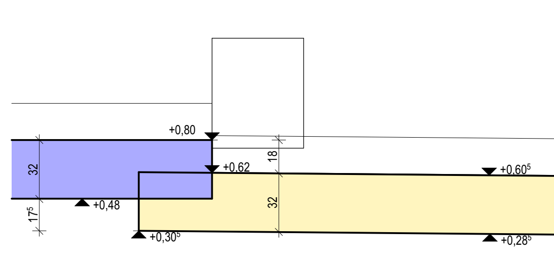
UG Übersicht Deckenversprünge Pausenhalle M1:100
