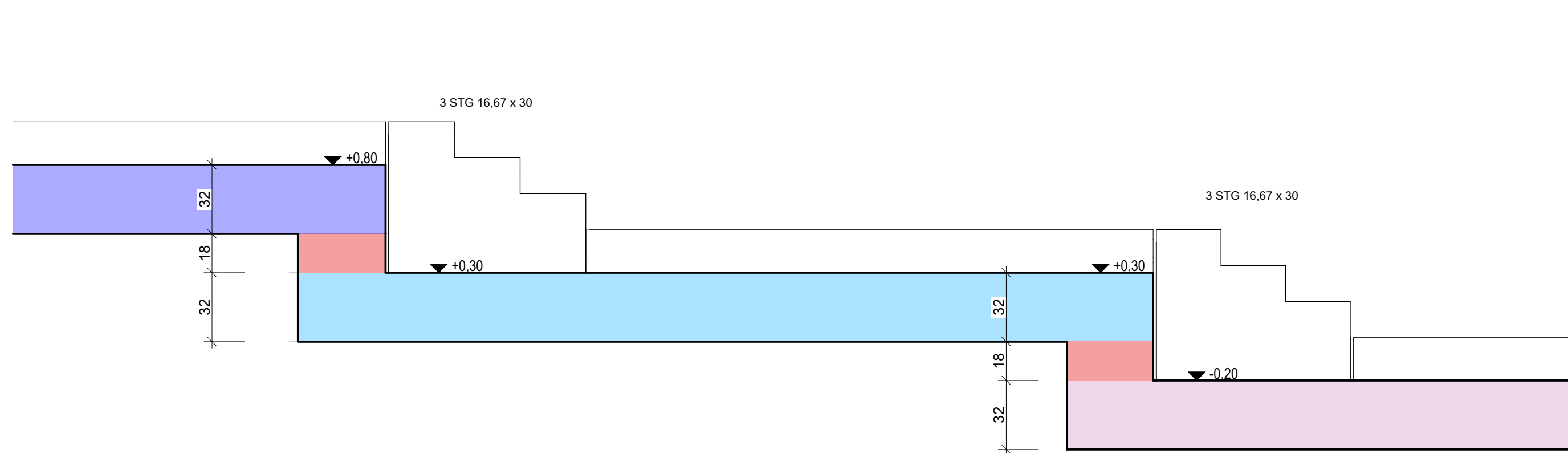
EG Übersicht Deckenversprünge Pausenhalle M1:100
