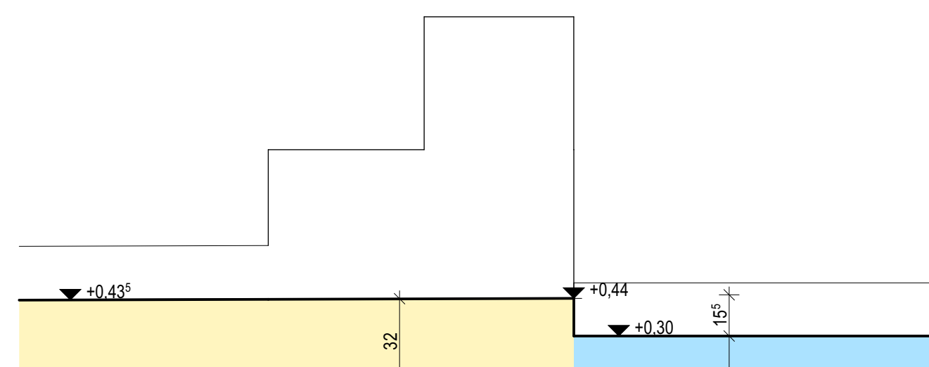
Z.9 Schnitt Zwischenpodest Übergabg Bauteil C zu D
