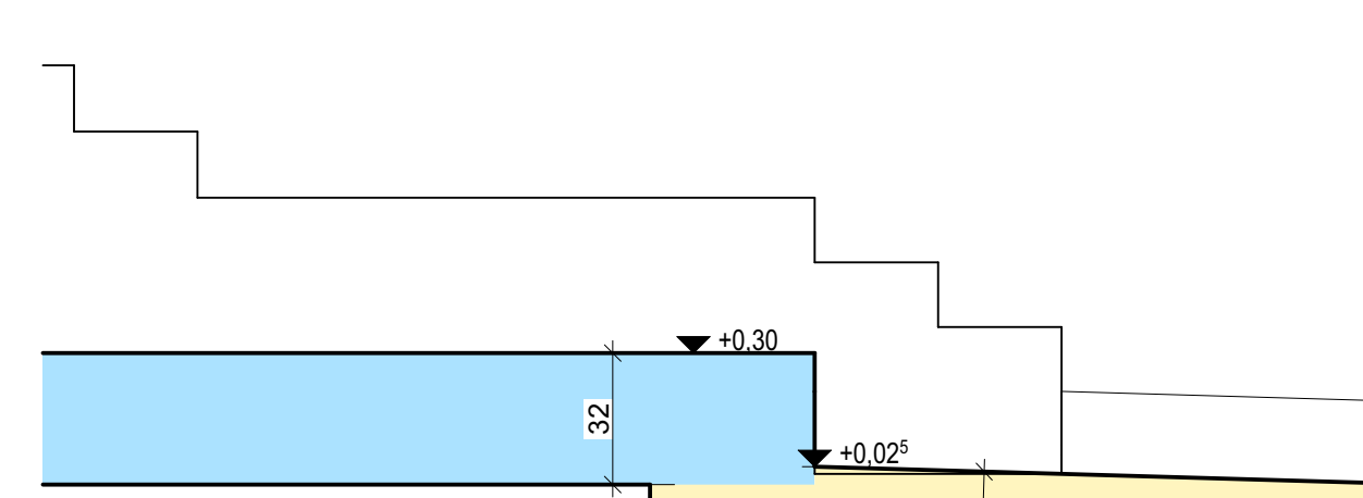
Z.6 Schnitt Podest Treppe Halle
