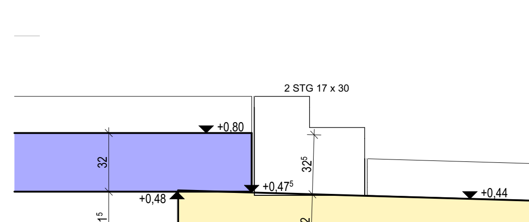
Z.3 Schnitt Treppe Bauteil A zu Bauteil B
