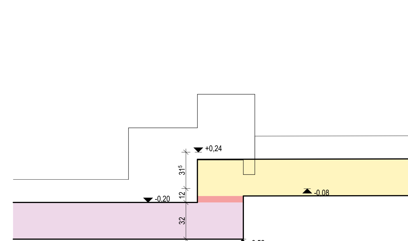
Z.11 Schnitt vor Bauteil C
