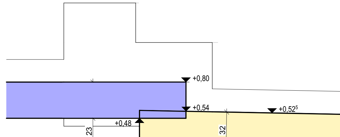
Z.2 Schnitt vor Bauteil A
