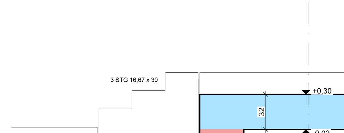
Z.7 Schnitt Treppe zu Mensa
