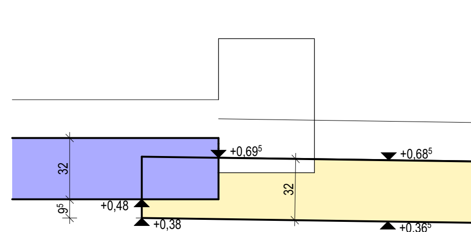
Z.1 Schnitt vor Bauteil A
