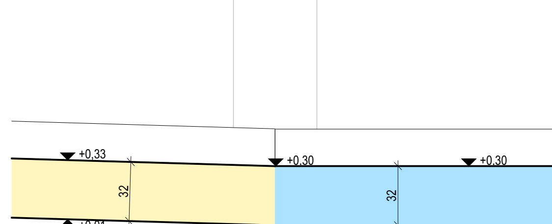
Z.4 Schnitt Barrierefreier Übergang Halle zu Bauteil B
