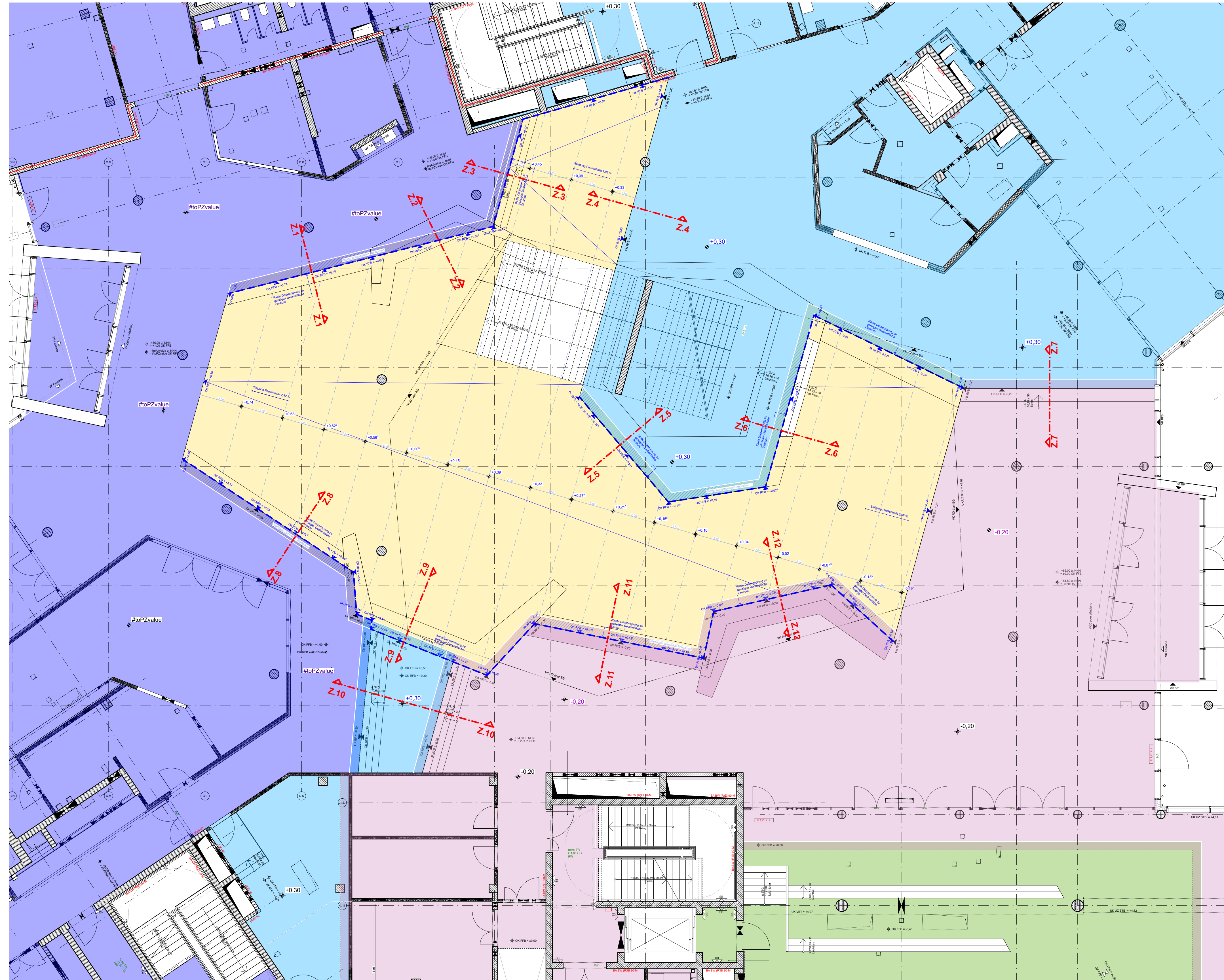
EG Übersicht Deckenversprünge Pausenhalle M1:100
