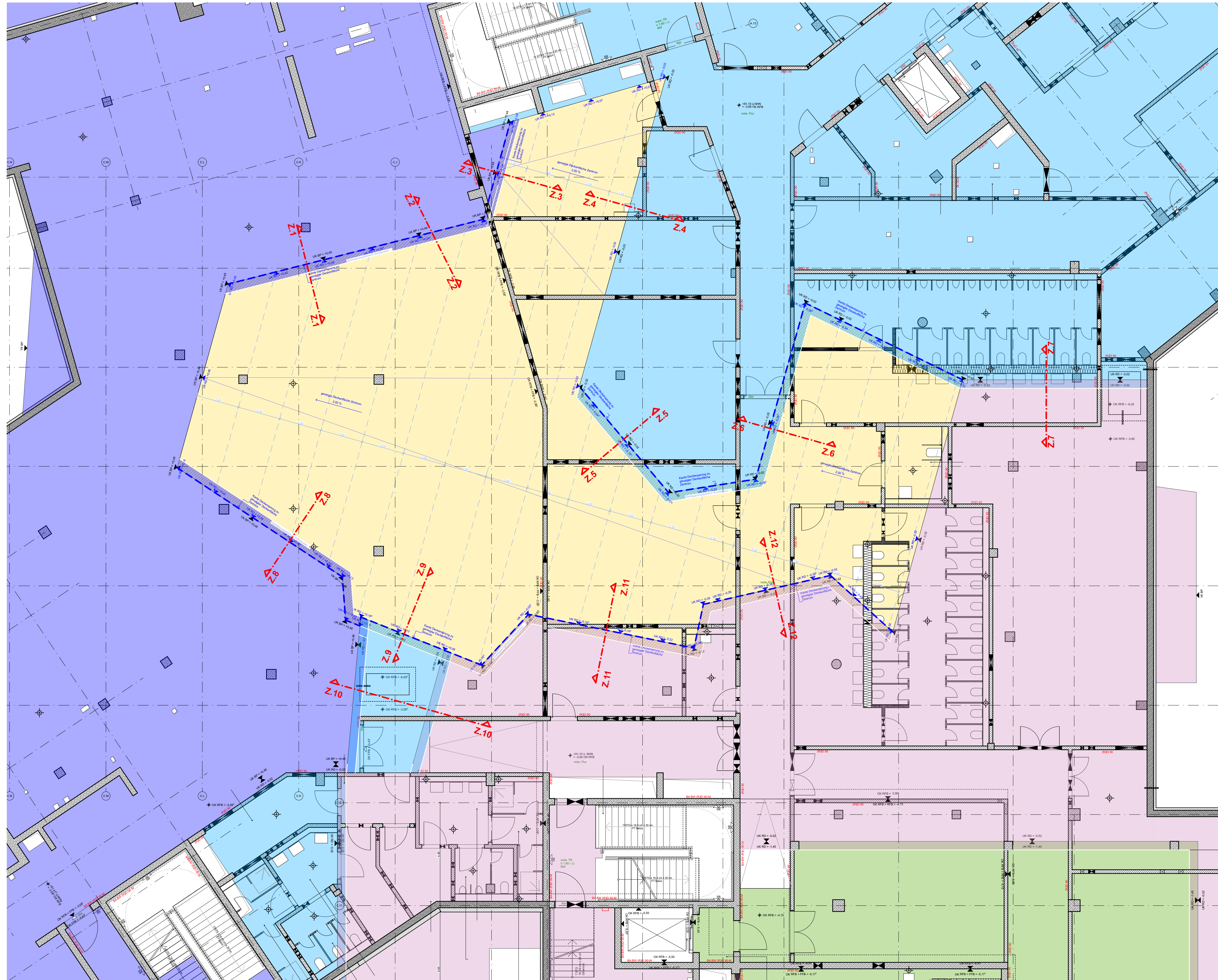
UG Übersicht Deckenversprünge Pausenhalle M1:100
