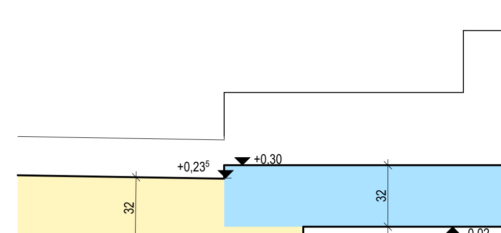
Z.5 Schnitt Podest Treppe Halle
